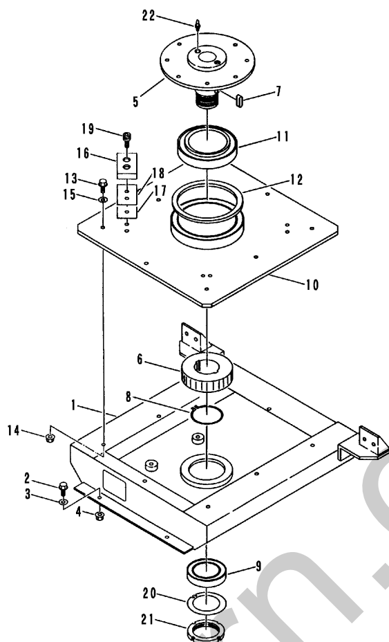
FIG 25 チュウカンフレーム (回転 & ダンプ) CENTER FRAME (SLEWING & DUMPING)
