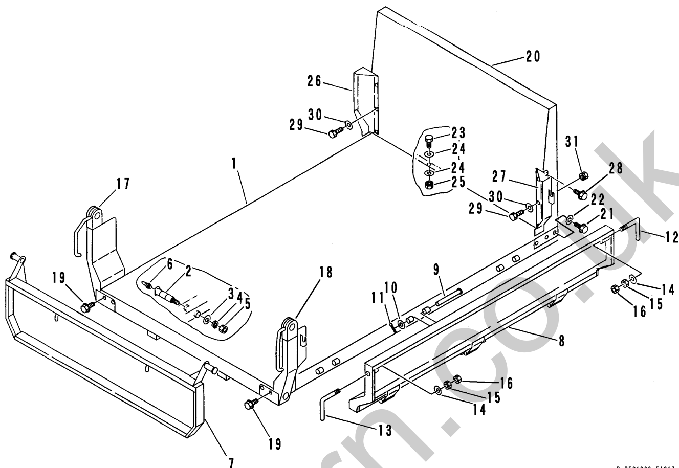
FIG 21 ニダイ & マエドア (一方ダンプ) WAGON & GATE (1-WAY DUMPING)
