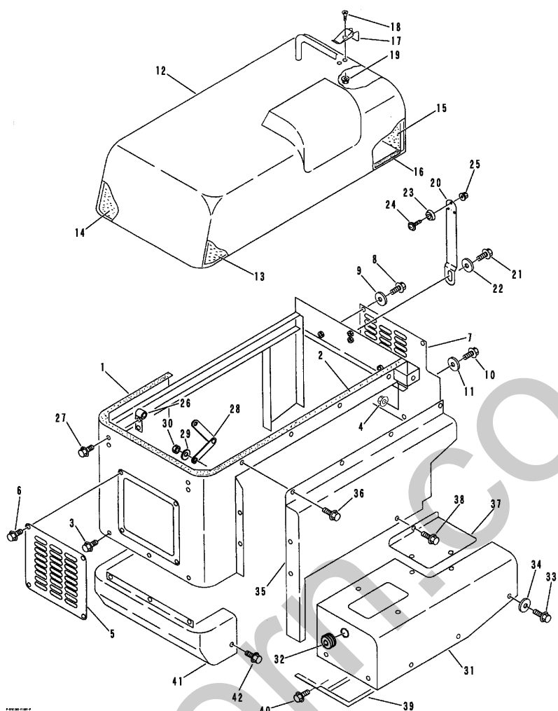
FIG 9 エンジンカバー ENGINE COVER
