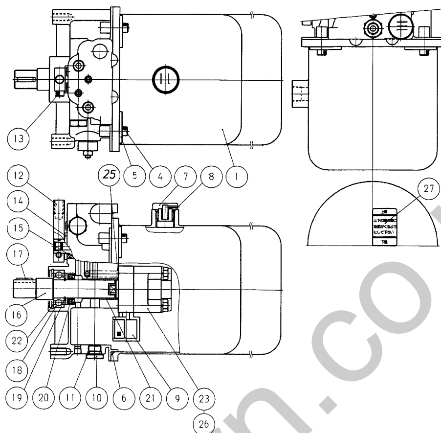
FIG 36 パッケージ (三転ダンプ・一方ダンプ) HYDRAULIC PUMP NO.6340434～
