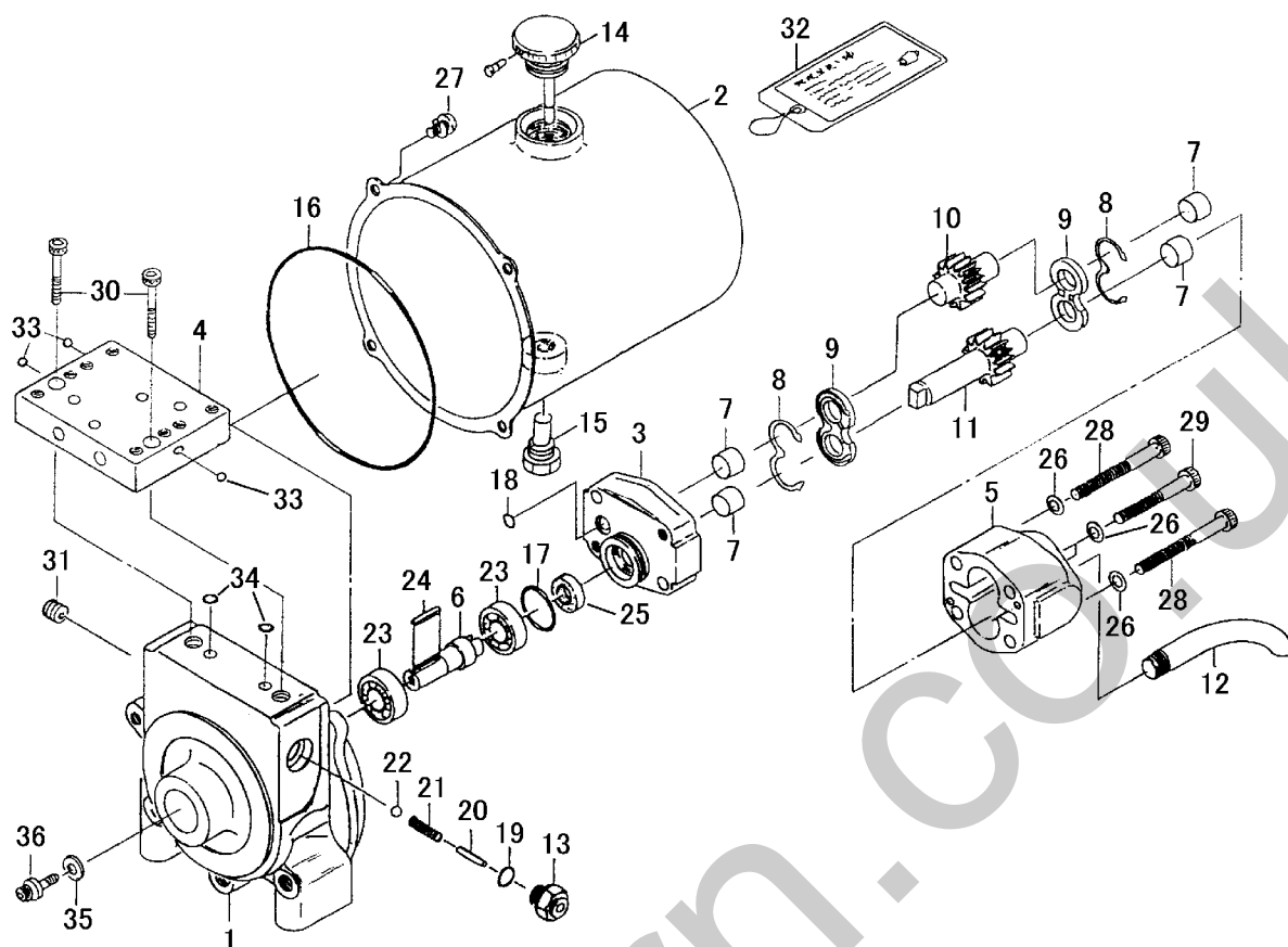
FIG 38 ユアツパッケージ (ソノ1) (ターン&ダンプ) HYDRAULIC PUMP (PART-1) (SLEWING&DUMPING)
