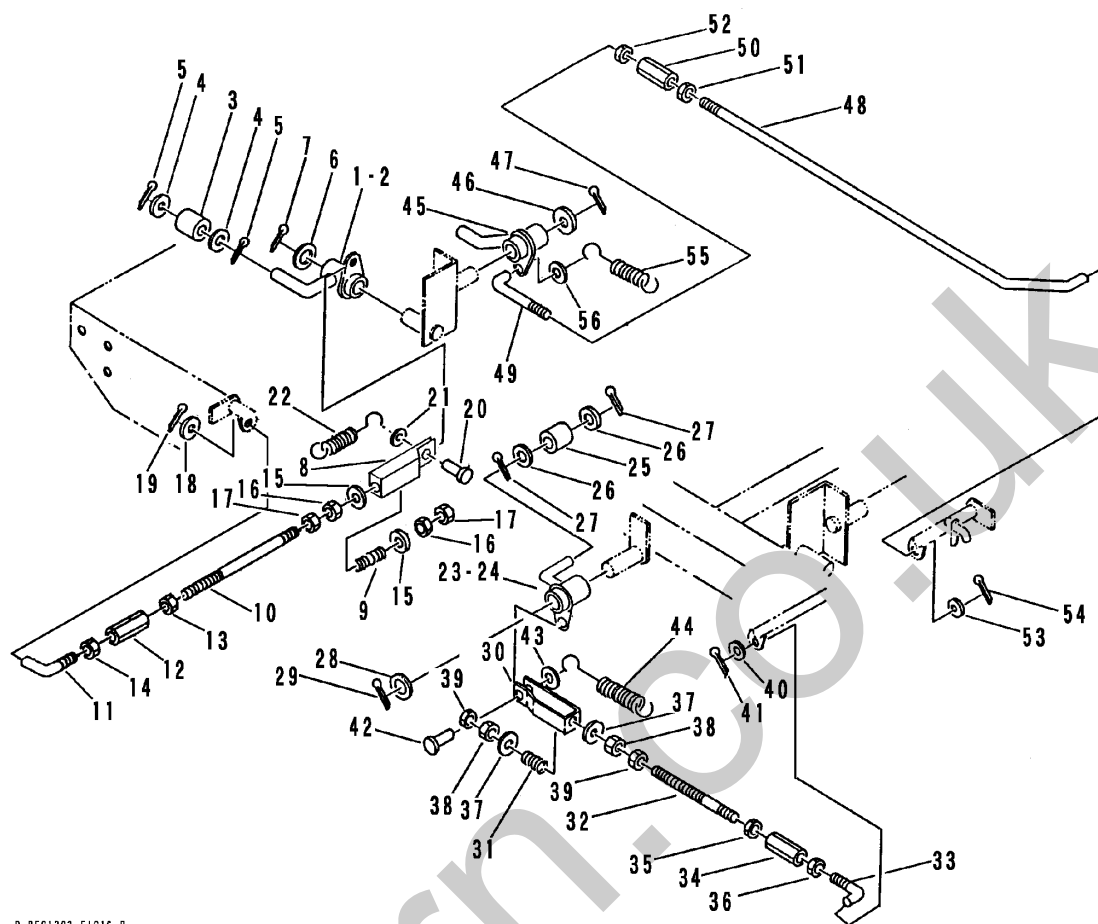
FIG 20 ドアロック (三転ダンプ) DOOR LOCK (3-WAY DUMPING)
