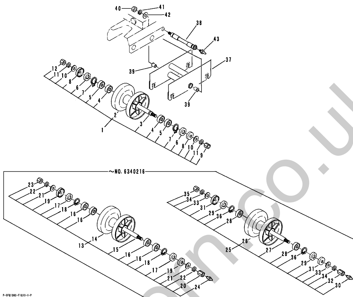
FIG 12 テンリン (国内用) ROLLER &amp; IDLER (DOMESTIC)
