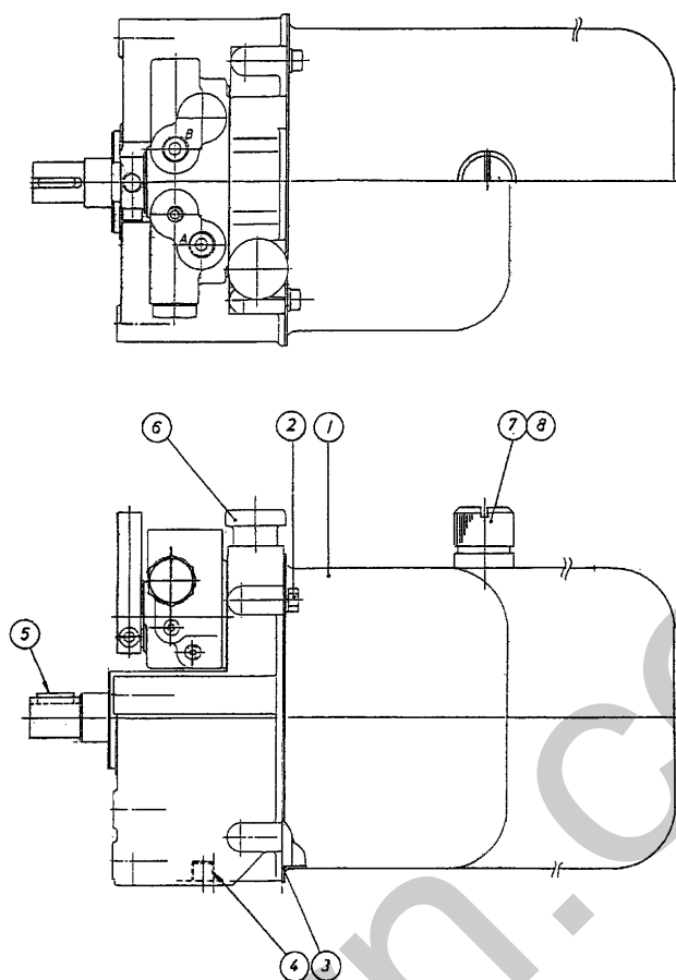
FIG 37 パッケージ (三転ダンプ・一方ダンプ) HYDRAULIC PUMP ~NO.6340433
