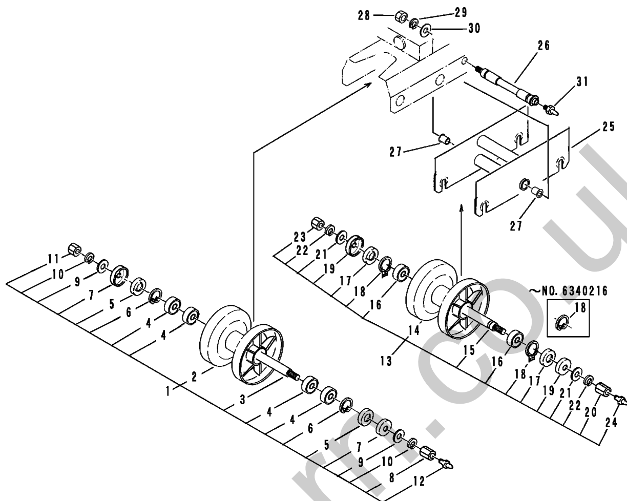
FIG 13 テンリン (輸出用) ROLLER (OVERSEAS)
