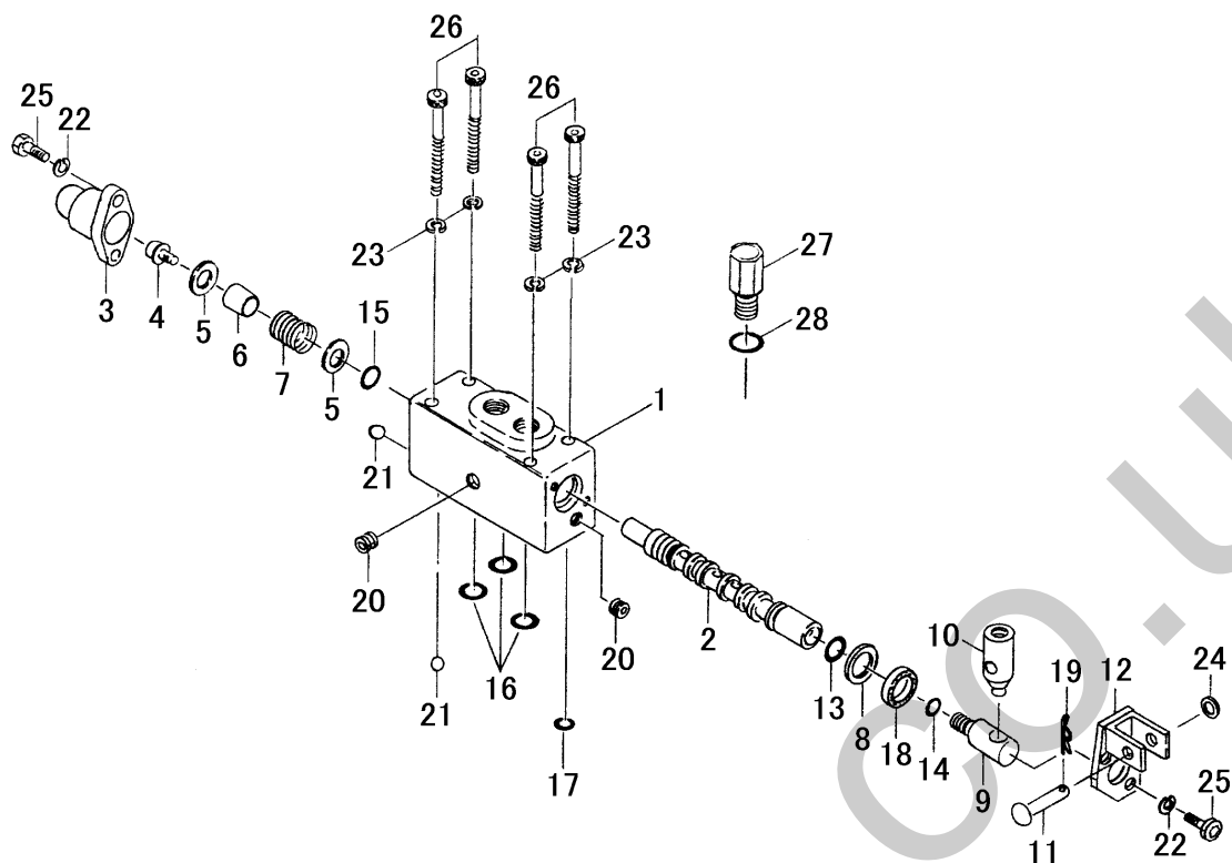
FIG 39 ユアツパッケージ (ソノ2) (ターン&ダンプ) HYDRAULIC PUMP (PART-2) (SLEWING&DUMPING)
