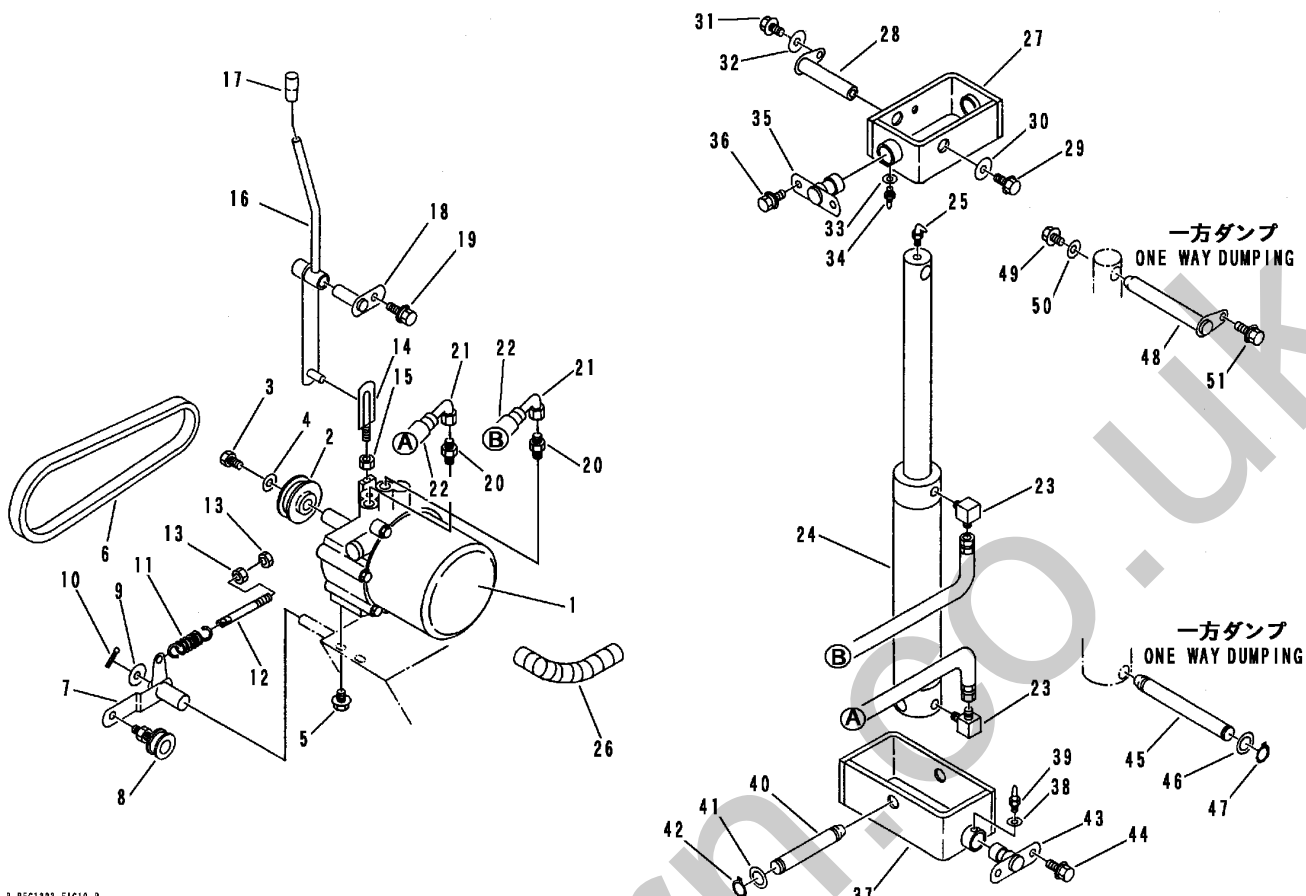
FIG 23 ハイドロリック システム (三転ダンプ・一方ダンプ) HYDRAULIC SYSTEM (3-WAY、1-WAY DUMPING)
