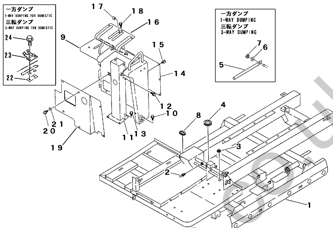
FIG 7 フレーム & ウンテンセキ FRAME & OPERATOR CAB
