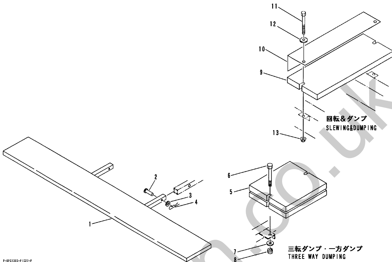
FIG 31 サイドボード & ウェート BORD & WEIGHT
