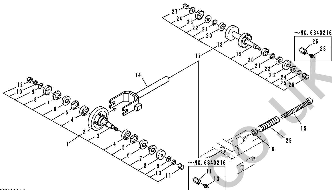
FIG 14 ユドウリン & シジテンリン (国内用) IDLER & ROLLER (DOMESTIC)
