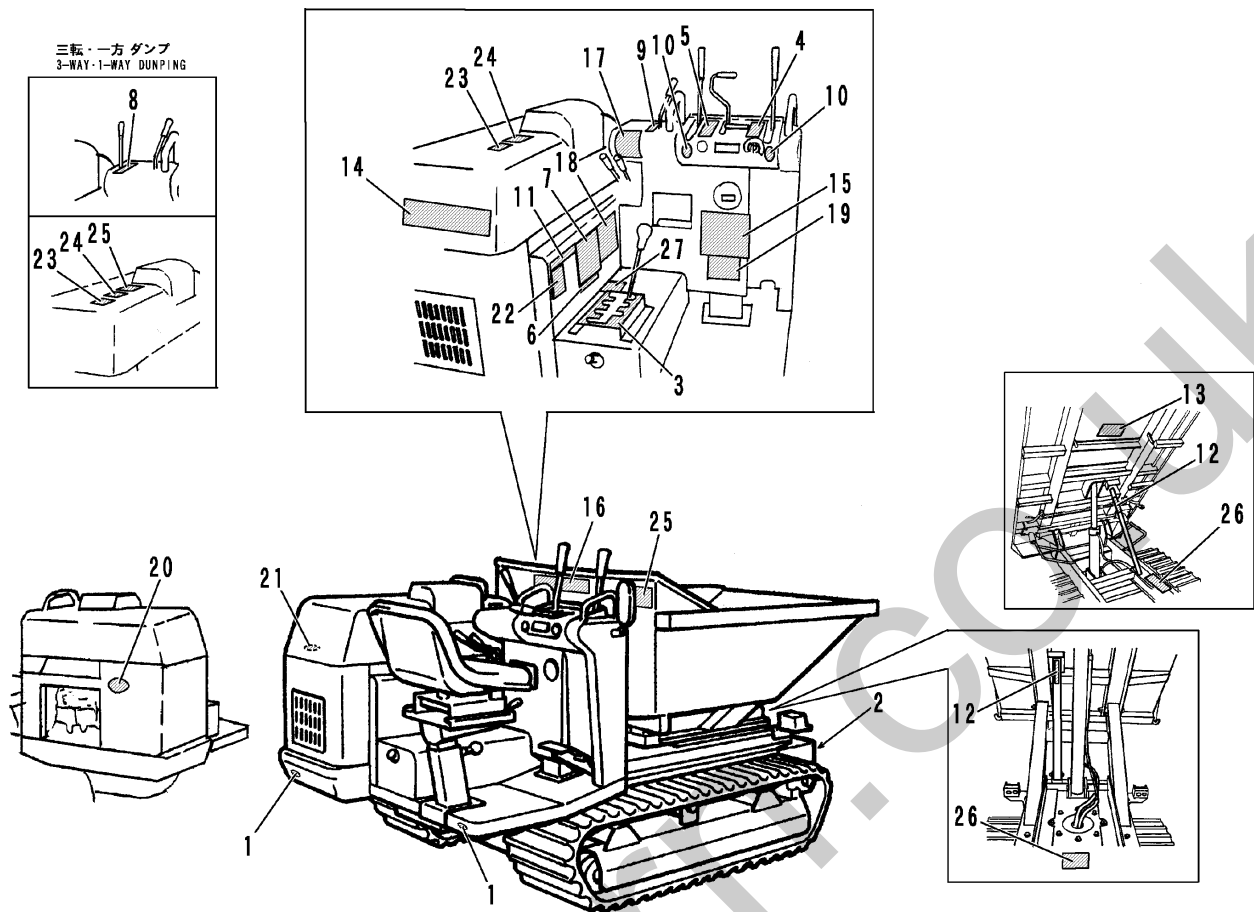
FIG 33 マーク (国内用) MARK (DOMESTIC)
