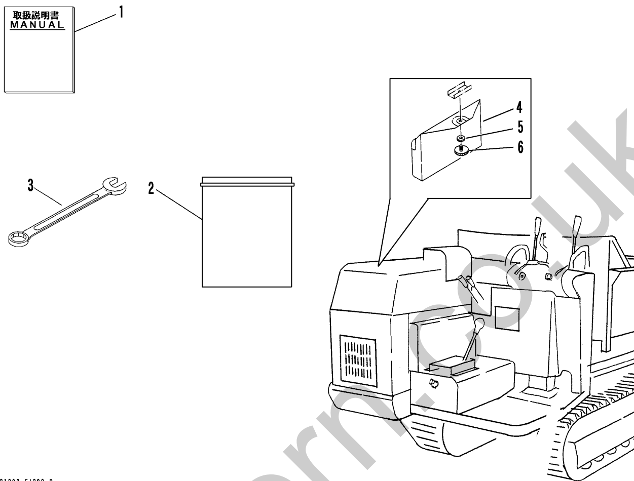
FIG 32 フゾクヒン ACCESSORIES
