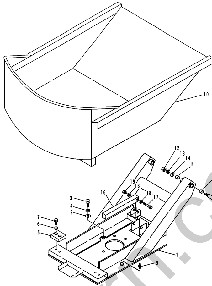
FIG 26 バケット & ターンテーブル (回転 & ダンプ) BUCKET & TURN TABLE (SLEWING & DUMPING)
