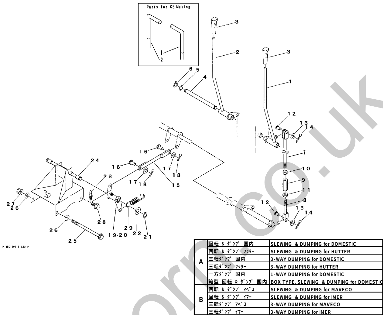
FIG 16 サイドクラッチレバー SIDE CLUTCH LEVER
