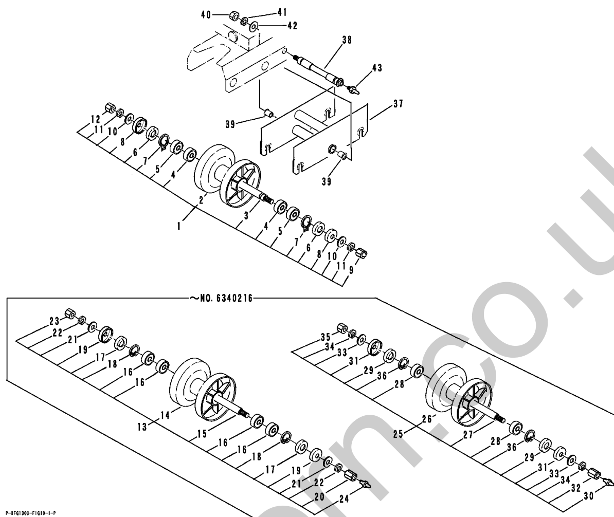
FIG 12 テンリン (国内用) ROLLER & IDLER (DOMESTIC)
