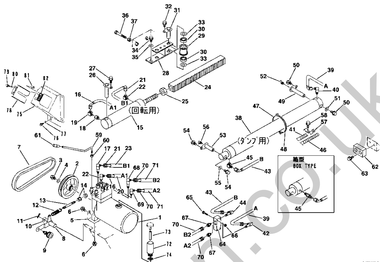
FIG 24 ハイドロリック システム (回転 & ダンプ) HYDRAULIC SYSTEM (SLEWING & DUMPING)
