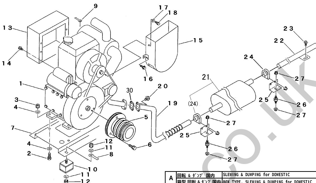
FIG 1 エンジン ENGINE
