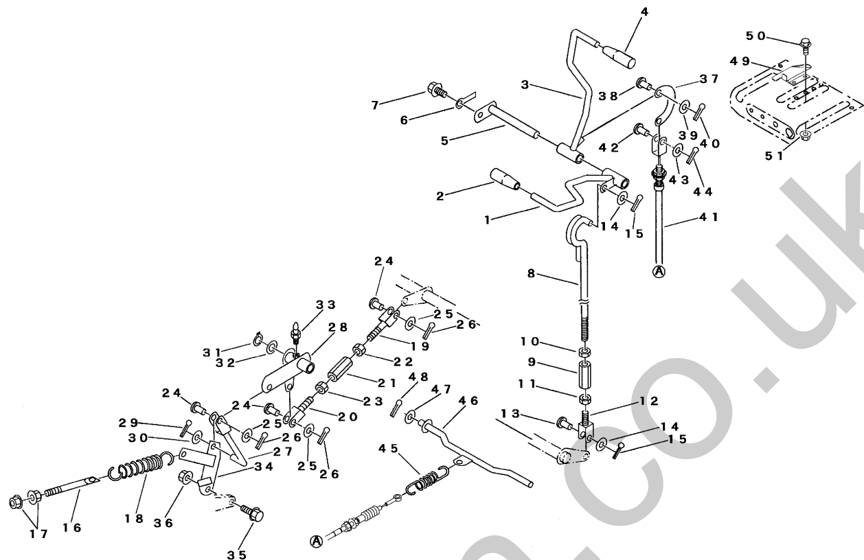
FIG 17 クラッチ & ブレーキレバー CLUTCH & BRAKE LEVER (～NO.6340400)
