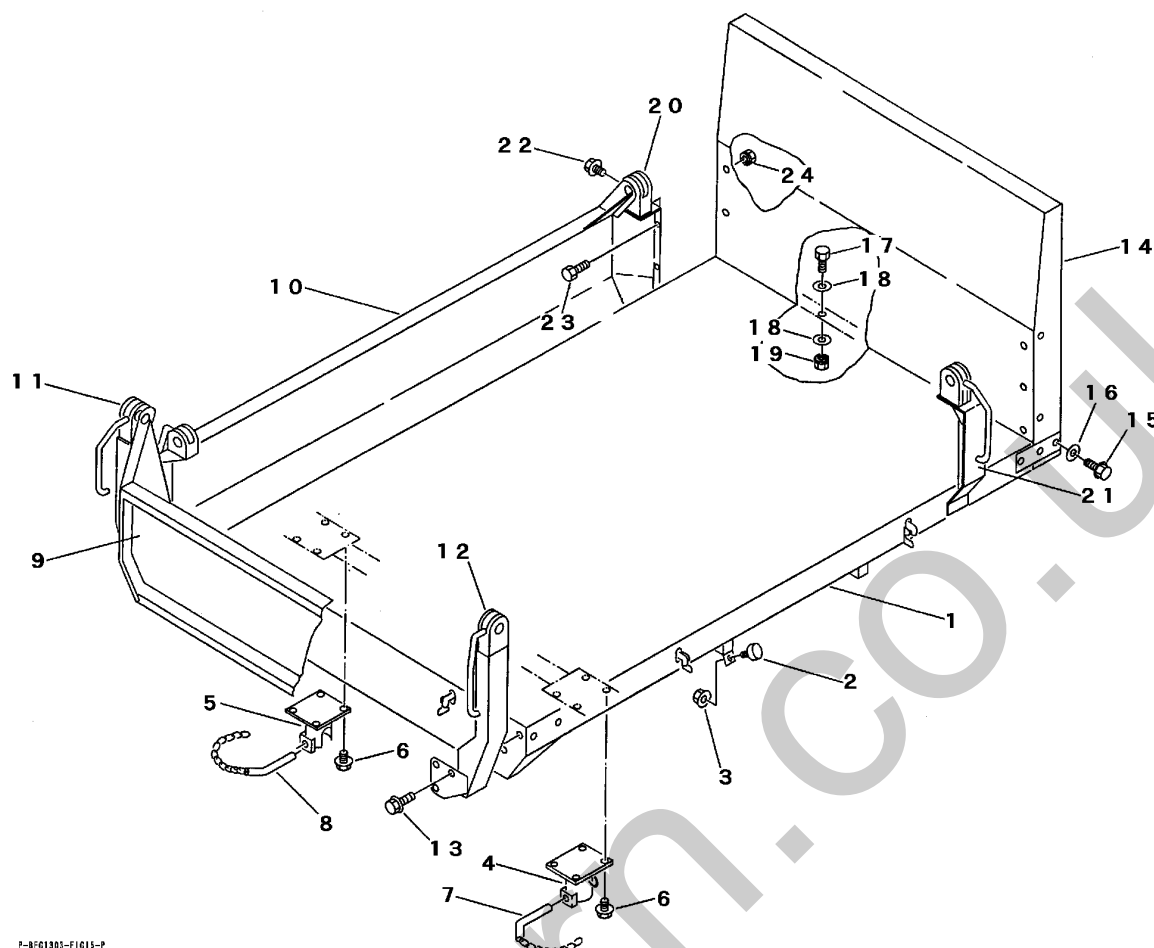
FIG 19 ニダイ & パネル (三転ダンプ) WAGON & PANEL (3-WAY DUMPING)
