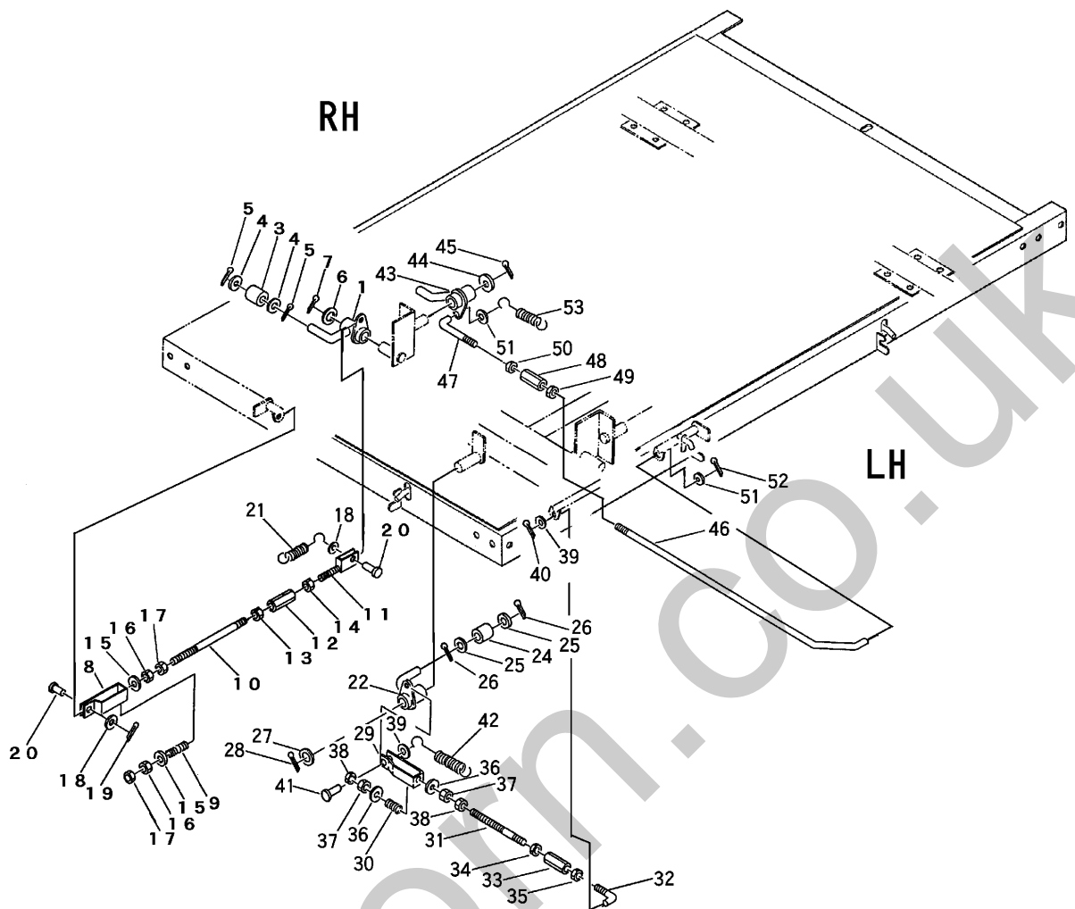
FIG 15 ドアロックソウチ DOOR LOCK (三転ダンプ)
