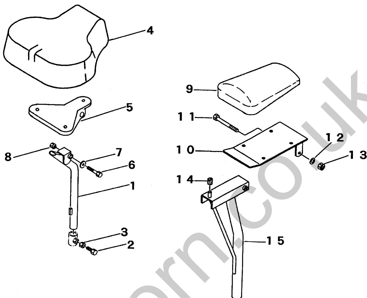
FIG 10 シート SEAT
