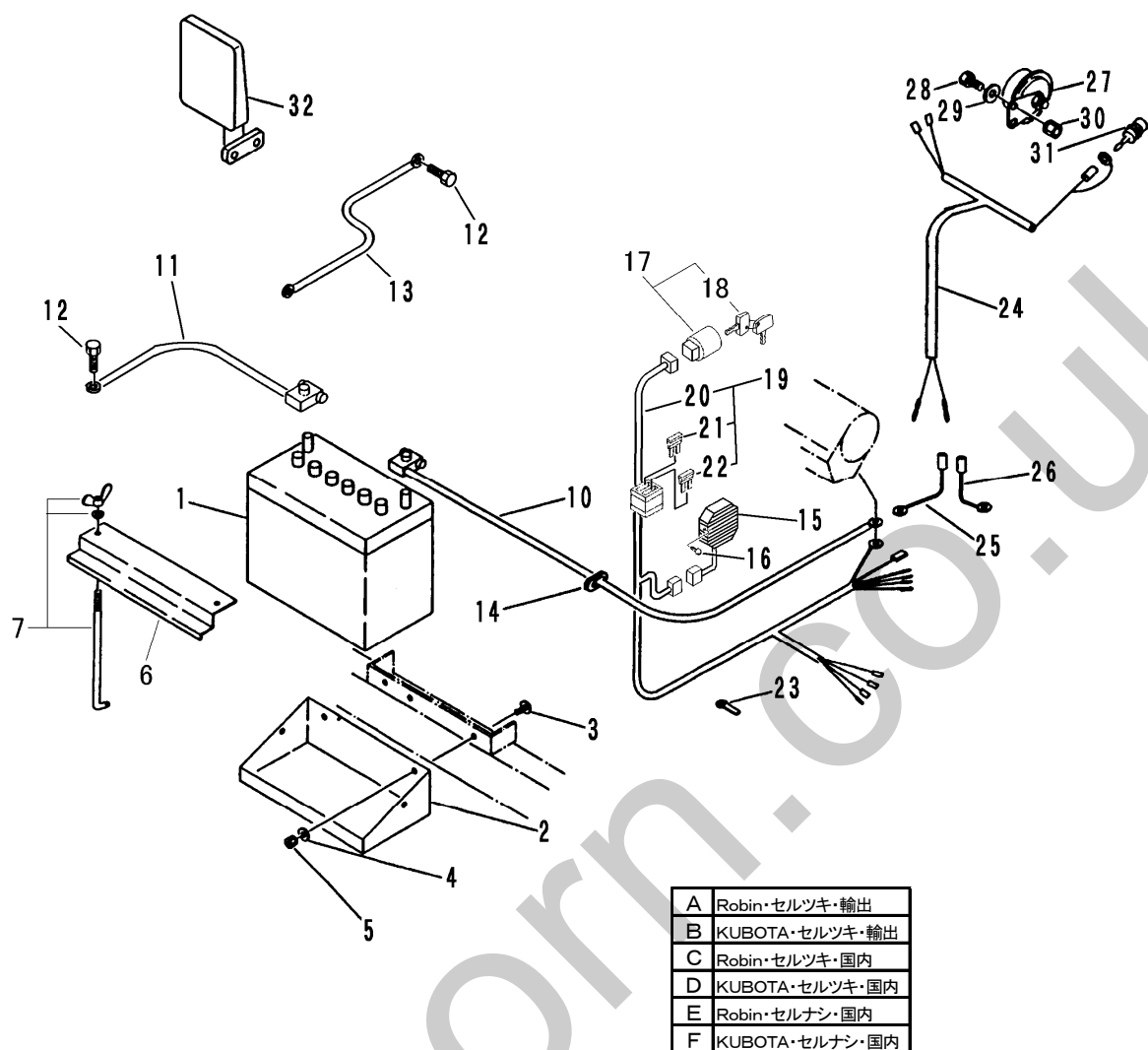
FIG 3 デンソウ ELECTRIC EQUIPMENT
