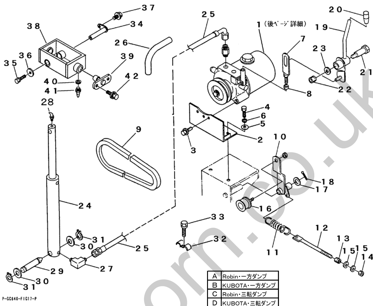
FIG 17 ユアツ HYDRAULIC
