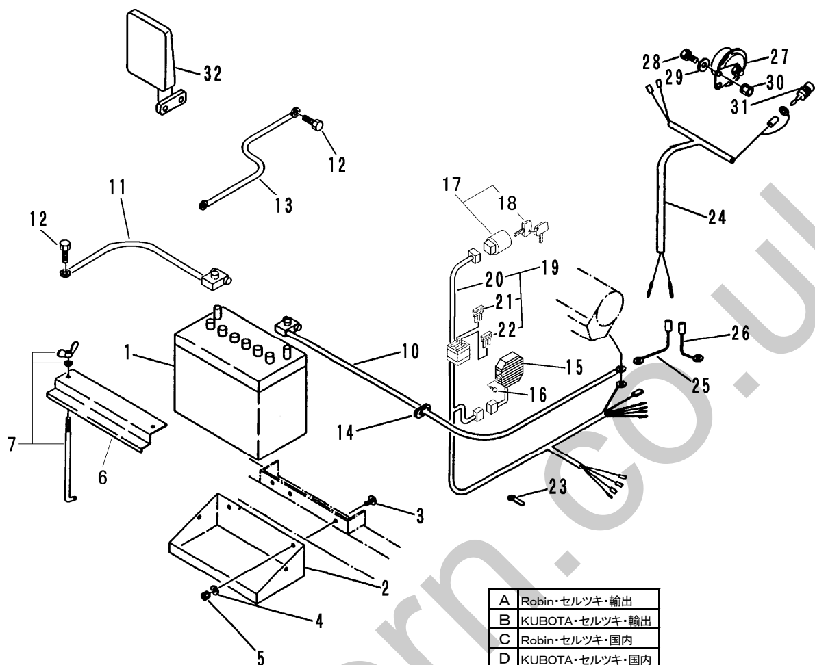
FIG 3 デンソウ ELECTRIC EQUIPMENT
