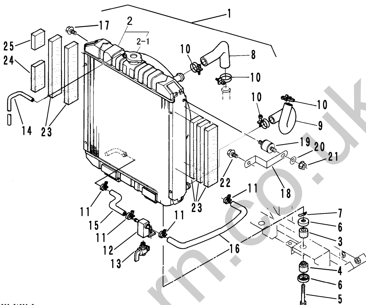
FIG 2 ラジエーター RADIATOR
