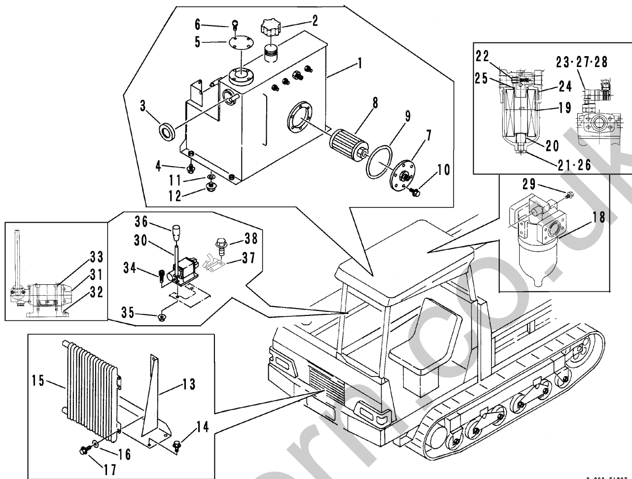
FIG 27 ユアツソウチ (ソノ1) HYDRAULIC SYSTEM (PART-1)
