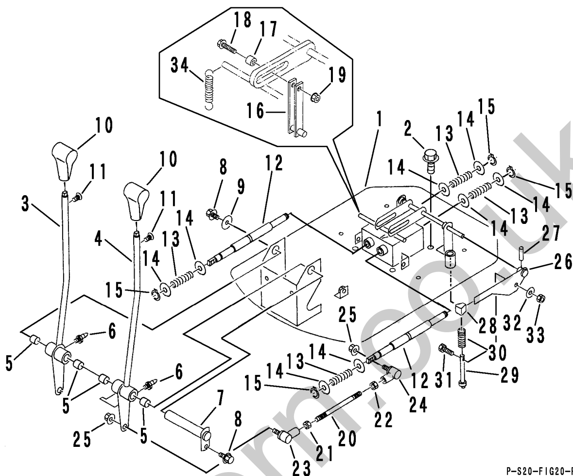
FIG 20 ステップ &amp; ソウコウレバー STEP &amp; LEVER
