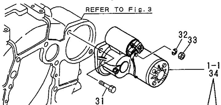
Fig. 15 スターティングモータ STARTING MOTOR
