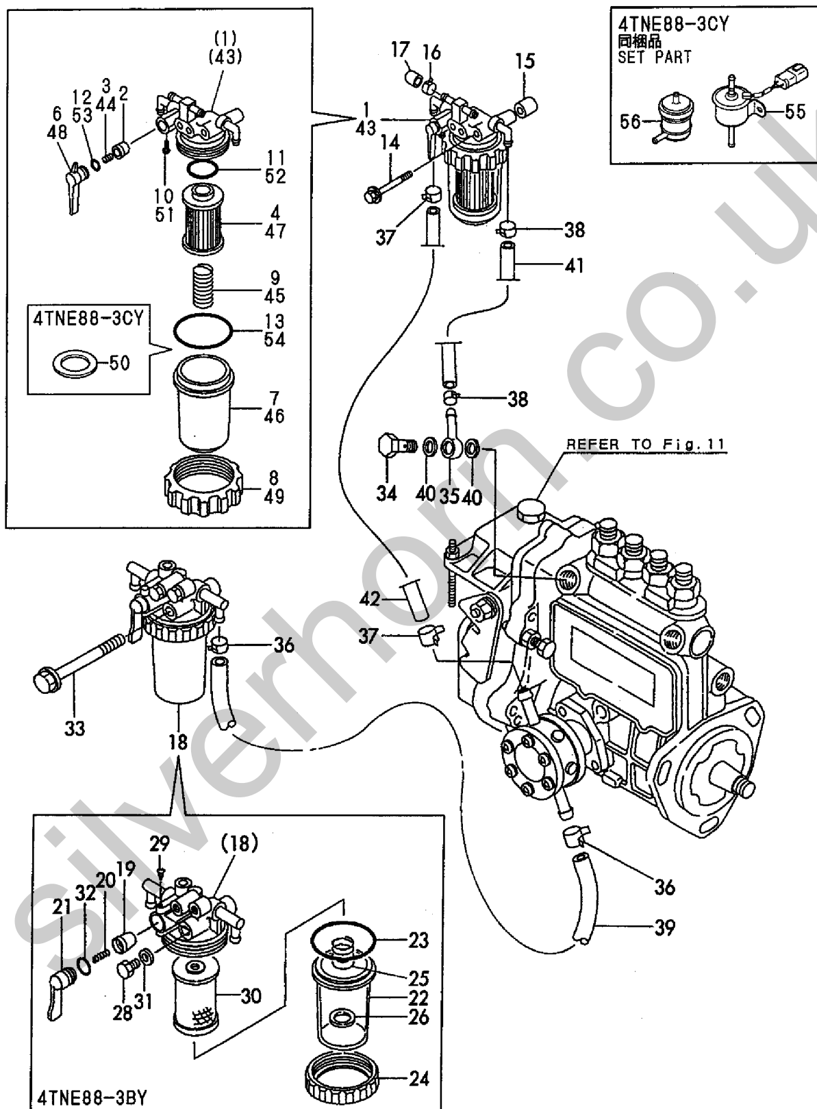
Fig. 14 燃料パイプ FUEL PIPE
