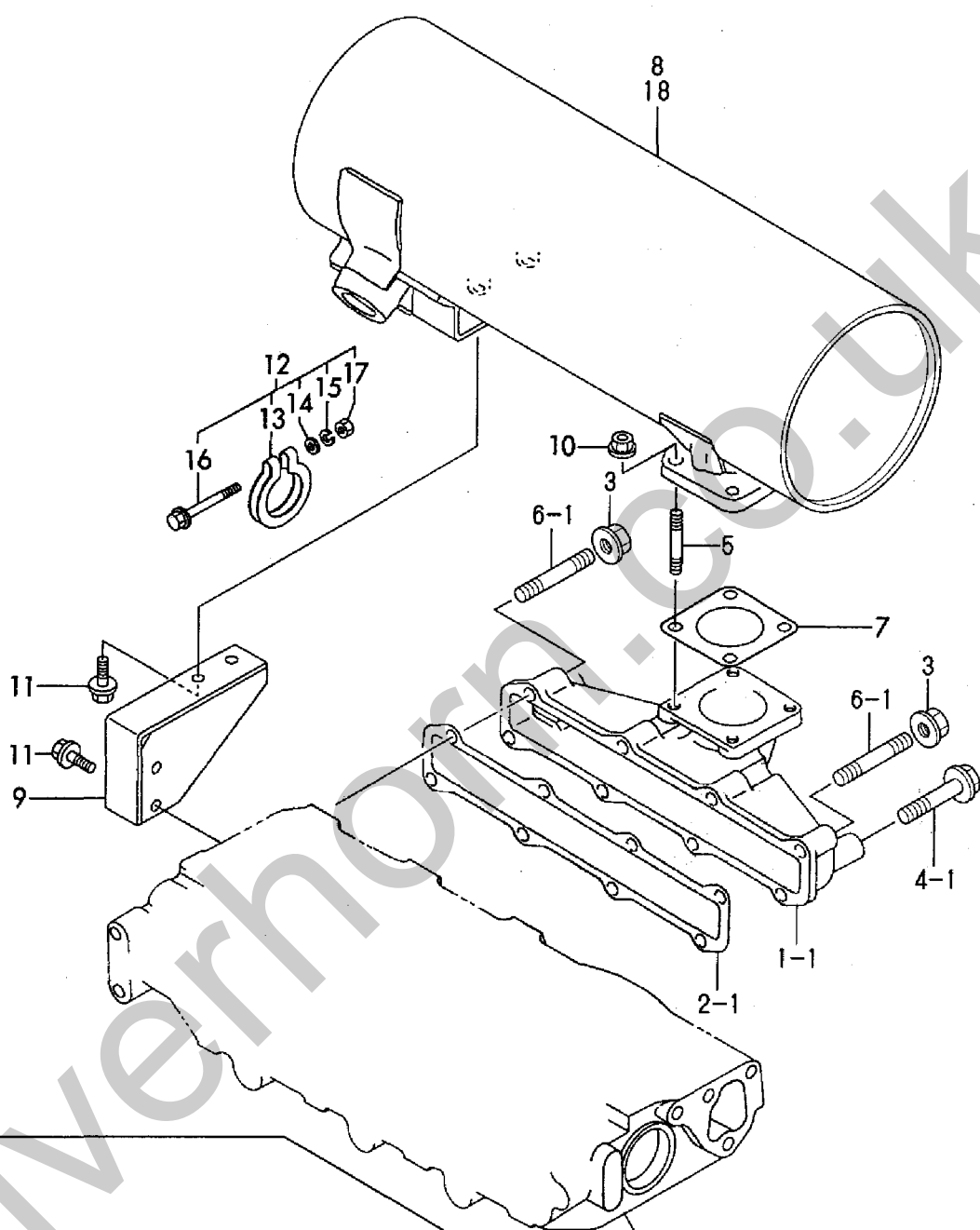
Fig. 6 排気マニホールド&サイレンサ EXH. MANIFOLD & SILENCER
