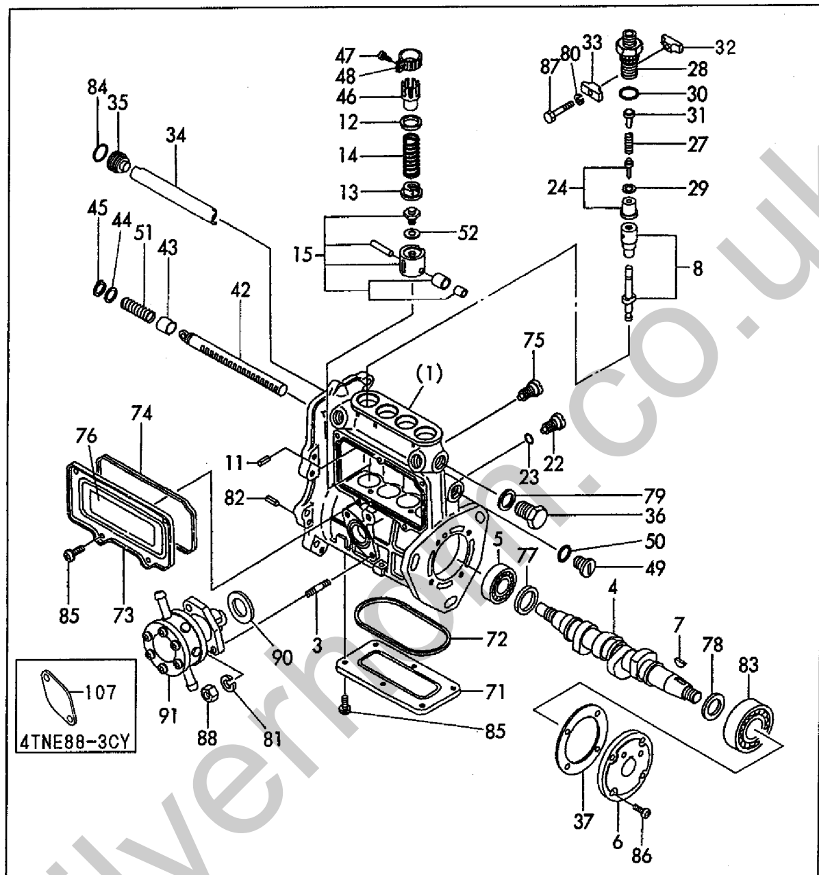
Fig. 11 燃料噴射ポンプ FUEL INJECTION PUMP
