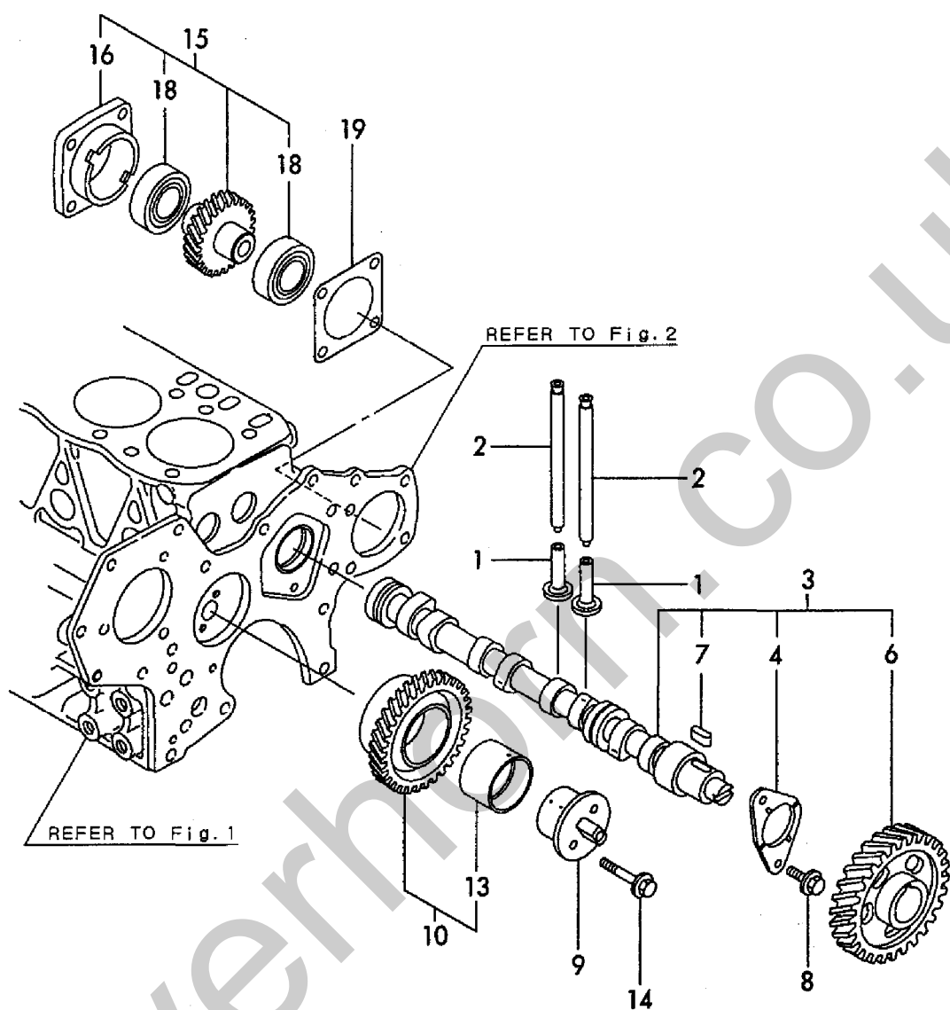
Fig. 7 カムシャフト & 駆動ギヤ CAMSHAFT & DRIVING GEAR
