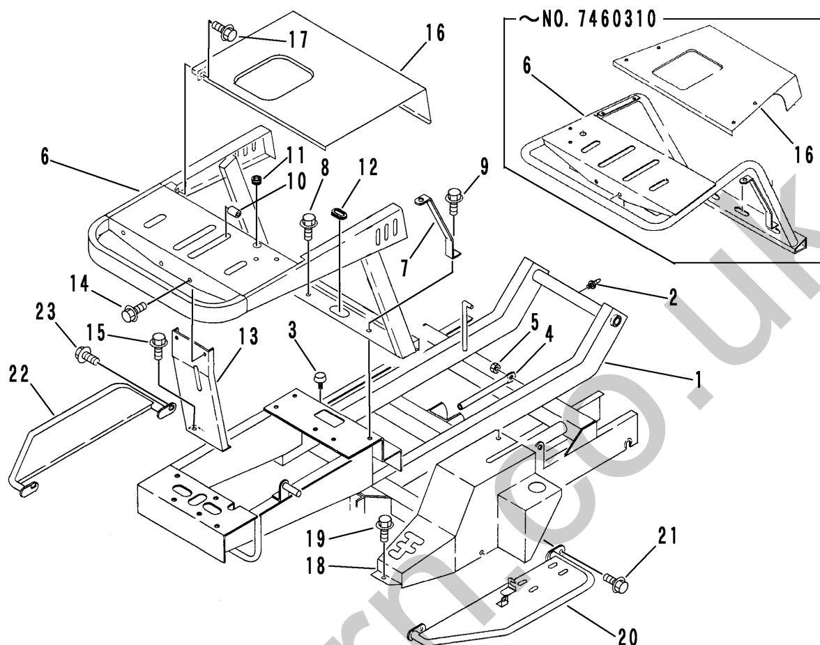
FIG 3 フレーム & エンジンカバー FRAME & ENGINE COVER
