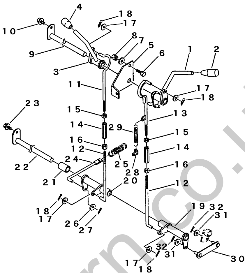
FIG 7 クラッチ &amp; ブレーキ CLUTCH &amp; BRAKE
