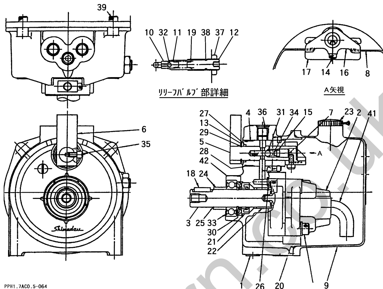
FIG 14 パッケージ HYDRAULIC PUMP
