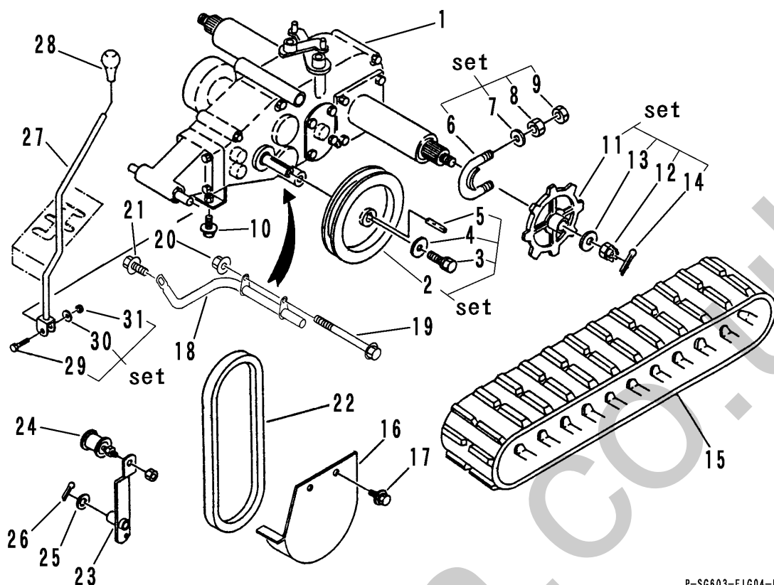
FIG 4 ミッション TRANSMISSION
