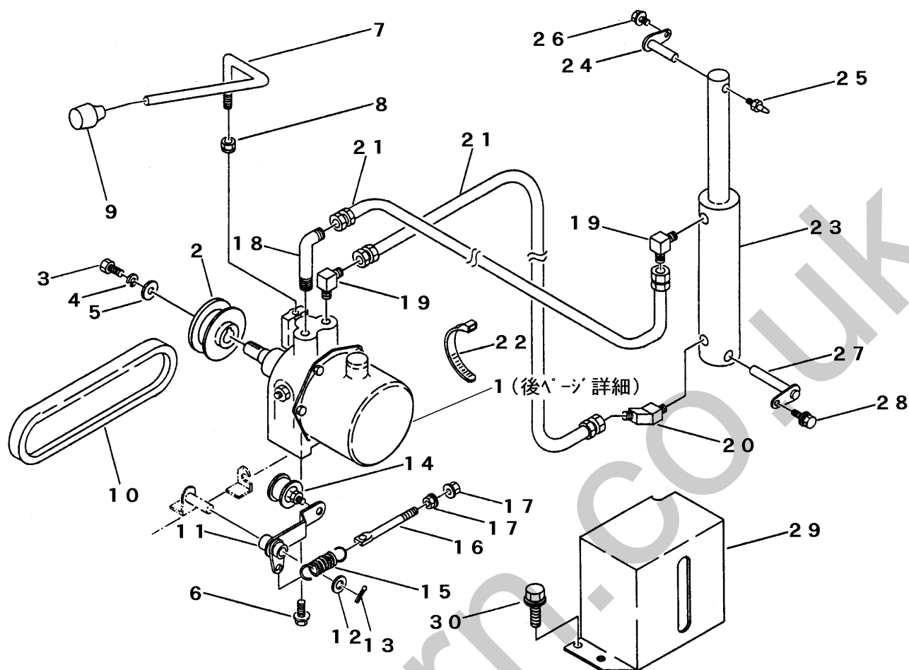
FIG 10 ユアツソウチ HYDRAULIC SYSTEM
