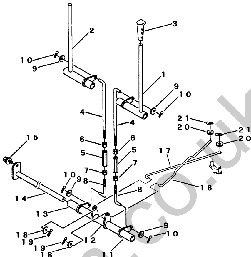
FIG 6 サイドクラッチ SIDE CLUTCH
