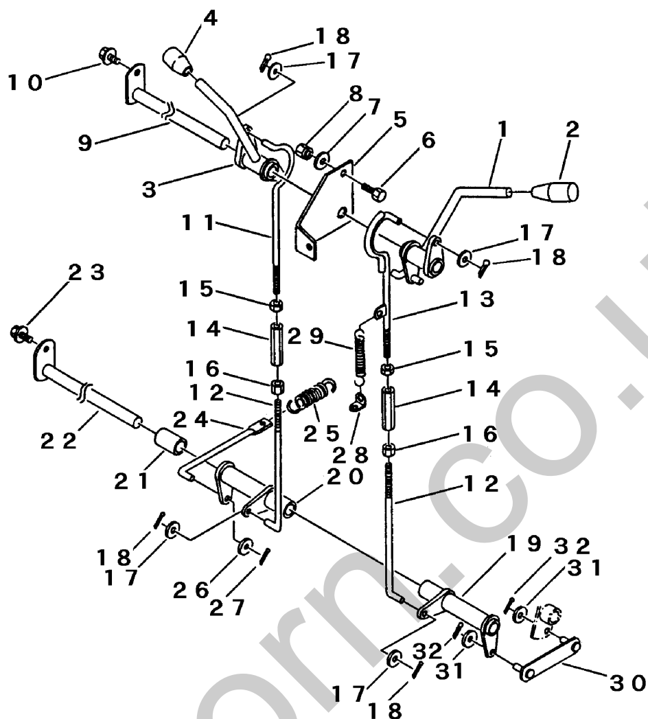
FIG 7 クラッチ & ブレーキ CLUTCH & BRAKE
