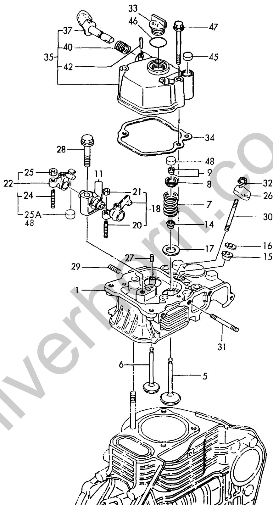
Fig. 2 シリンダヘッド&ボンネット CYLINDER HEAD & BONNET
