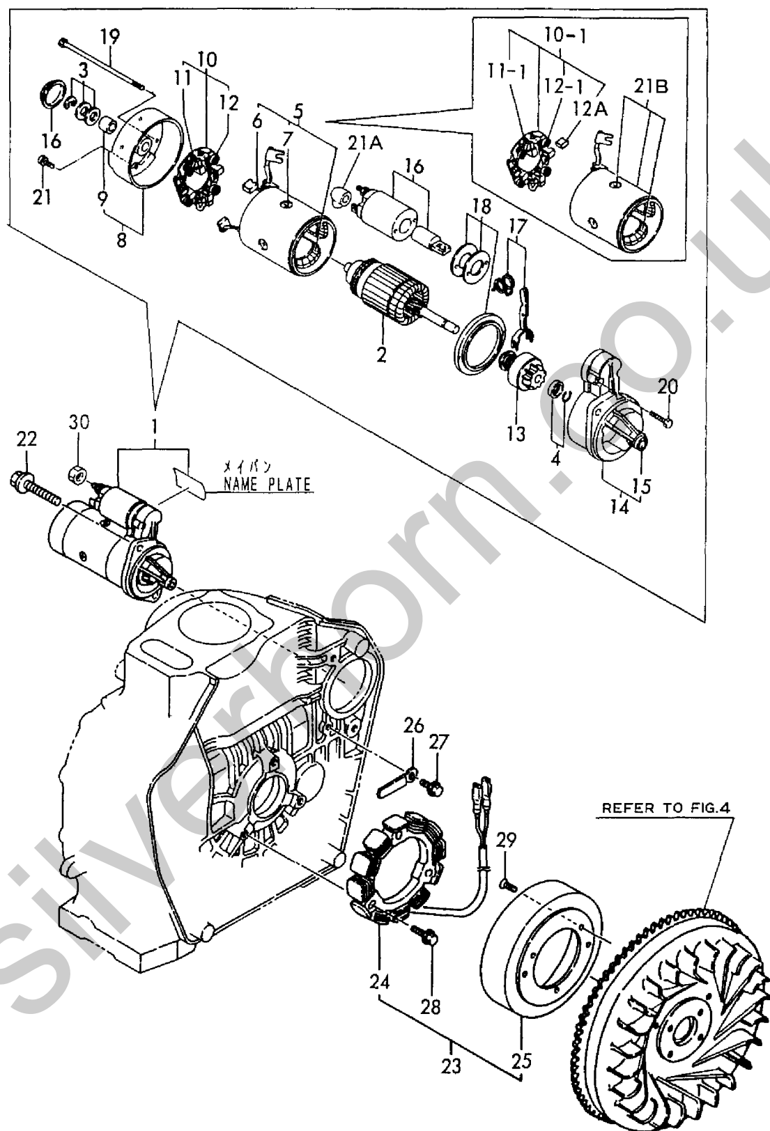
Fig. 9 スターティングモータ & ダイナモ STARTING MOTOR & DYNAMO
