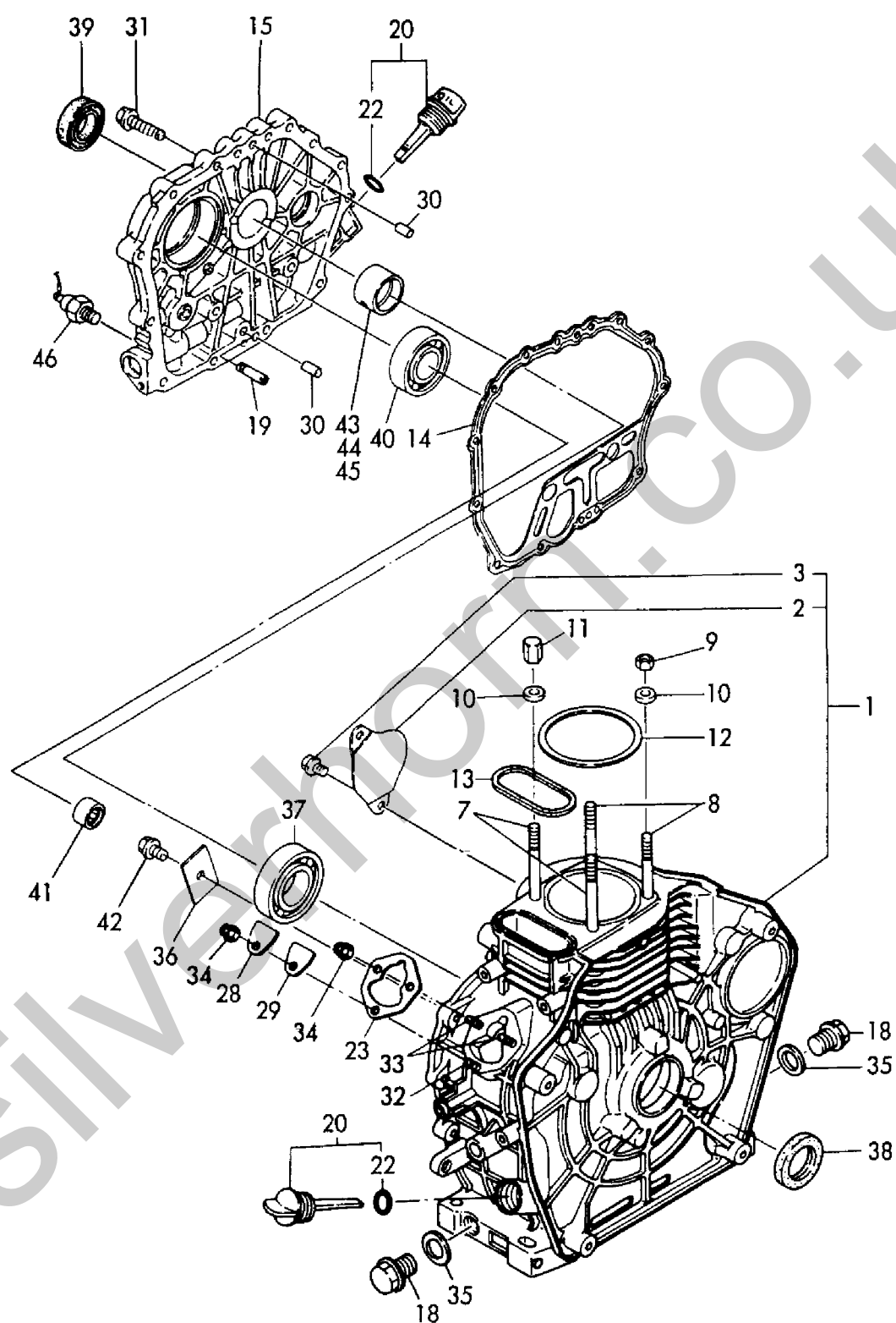
Fig. 1 シリンダブロック CYLINDER BLOCK
