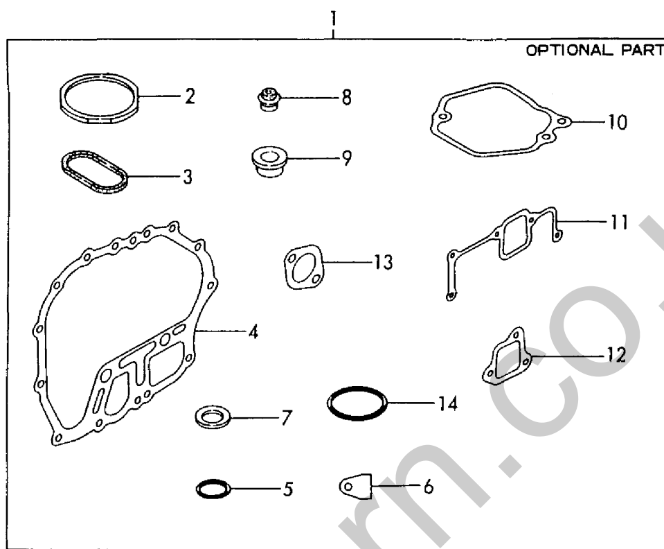
Fig. 10 パッキンセット(オプション) GASKET SET (OPTIONAL)
