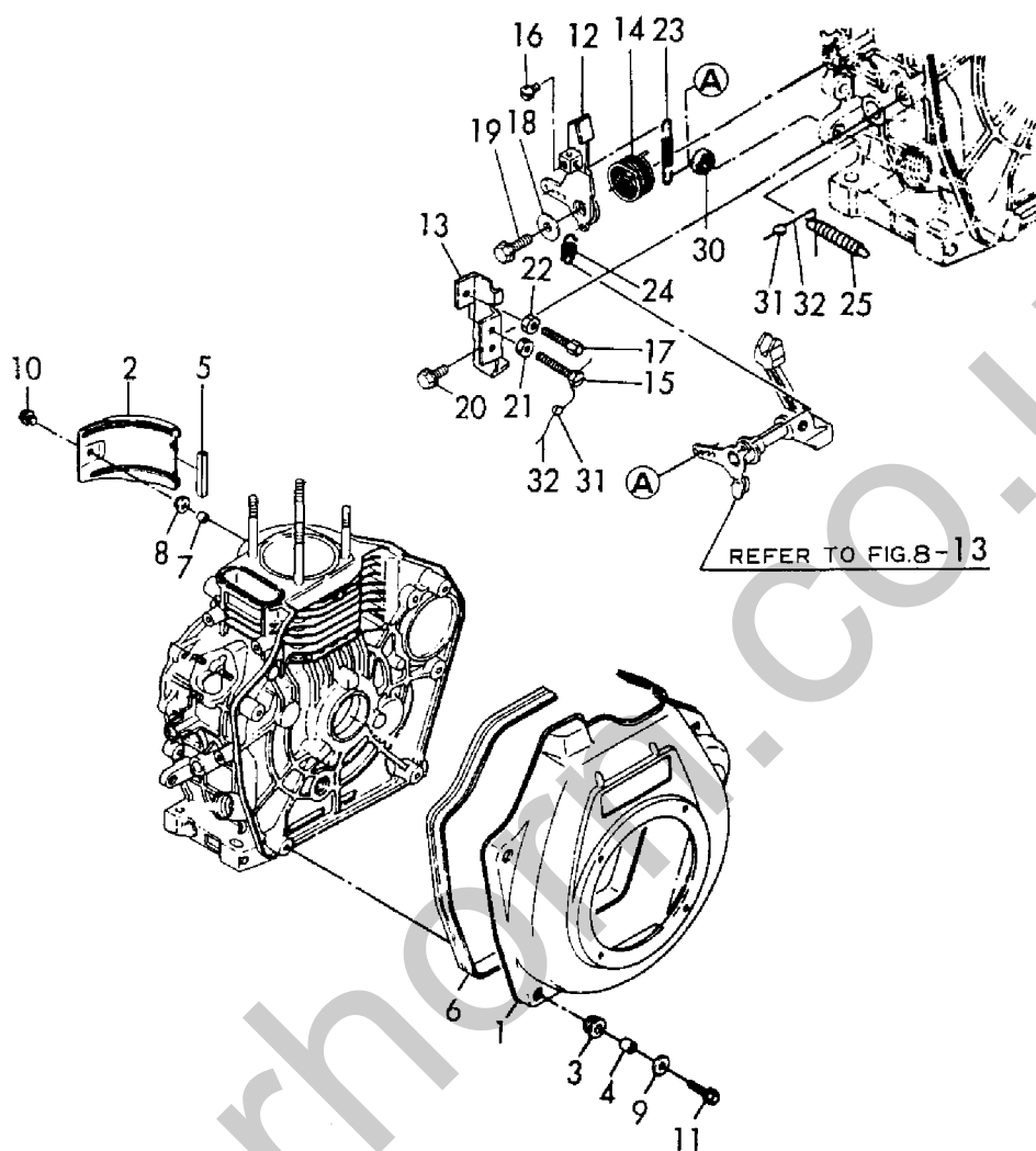
Fig. 5 レイキャク & シドウソウチ COOLING & STARTING DEVICE
