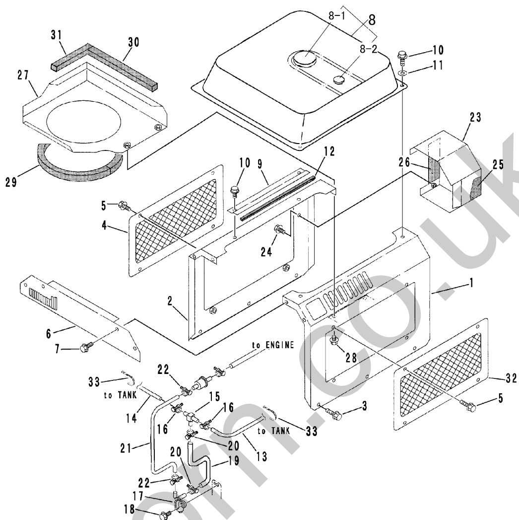
FIG 4 タンク TANK
