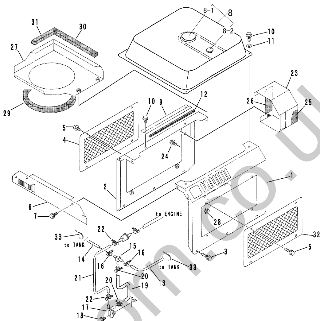
FIG 4 タンク TANK
