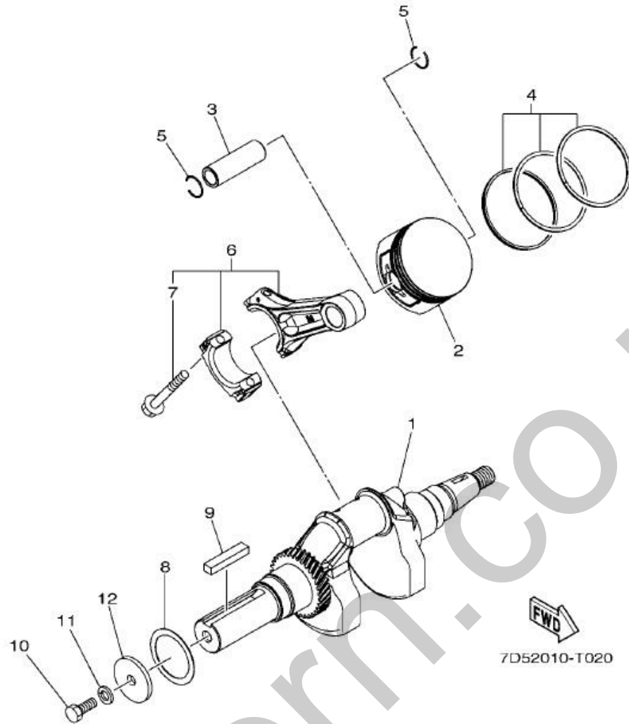
FIG. 2 クランクシャフト&ピストン CRANKSHAFT&PISTON
