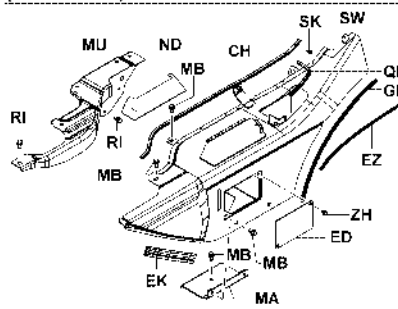
(STEEL CABIN)
