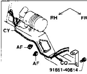
[FRAME RH SIDE,TANK]
