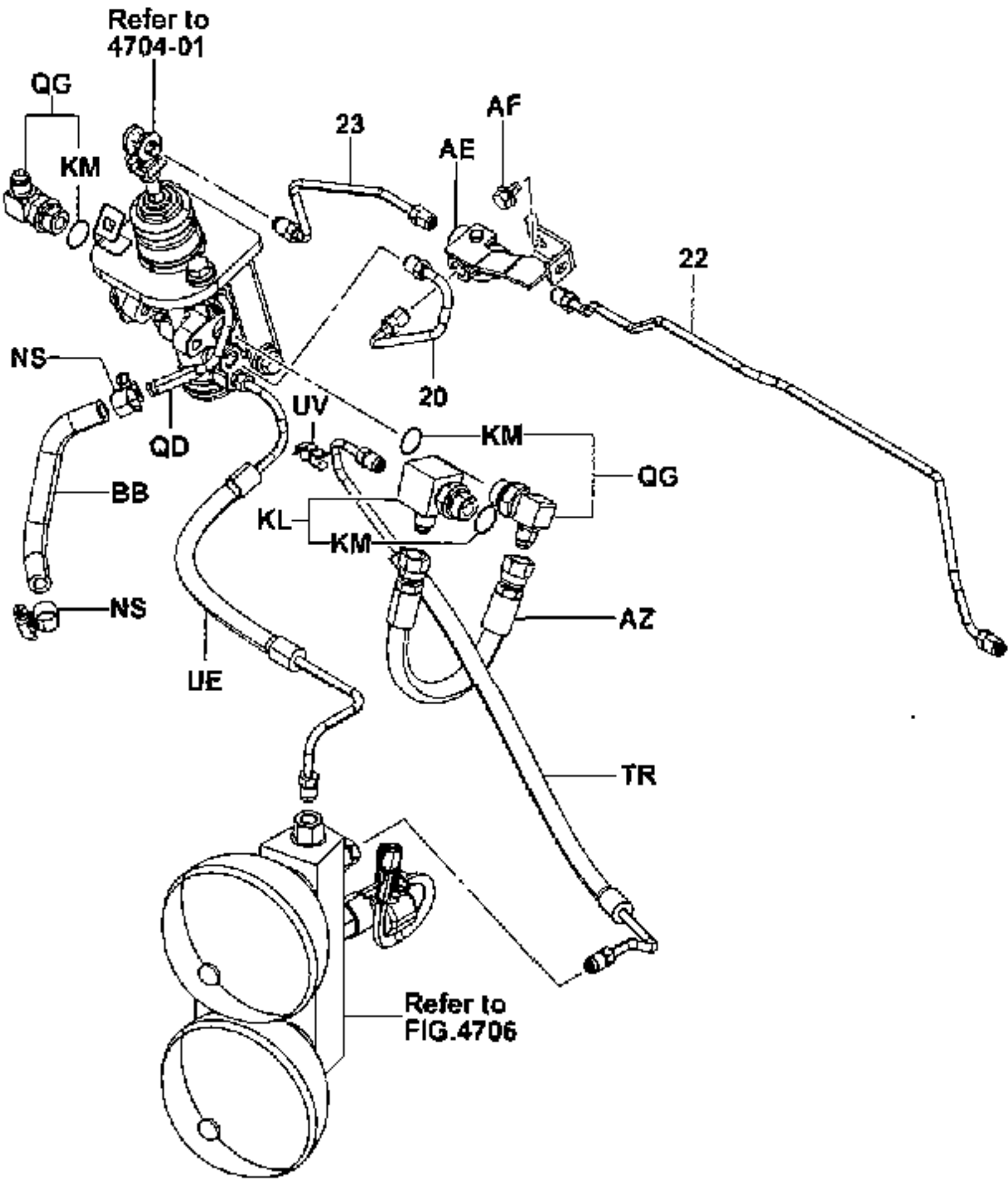
4714-269B
