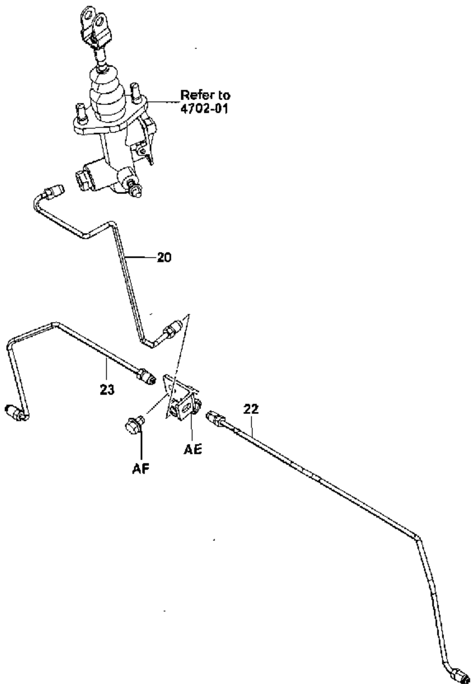
4714-268
