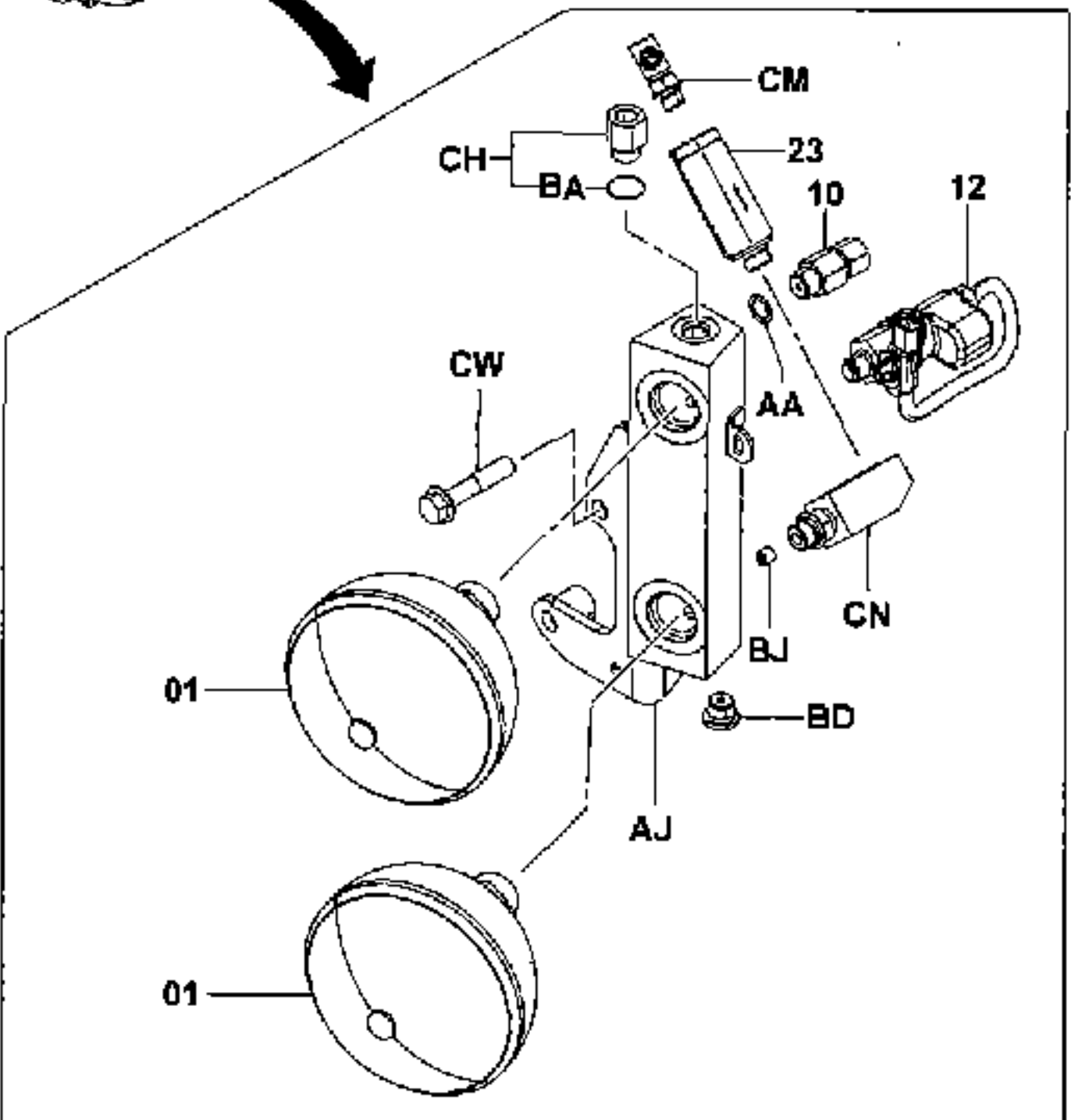
4706-021B
