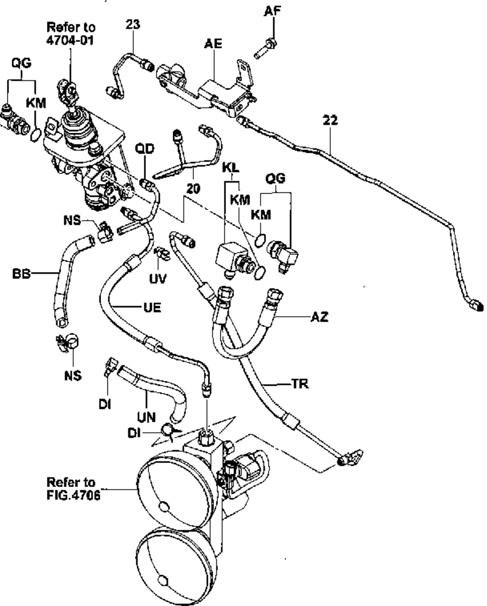
4714-273A
