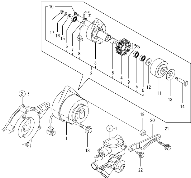
Fig.15. GENERATOR
