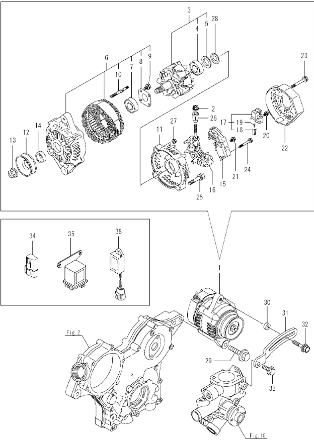
Fig.16. GENERATOR
