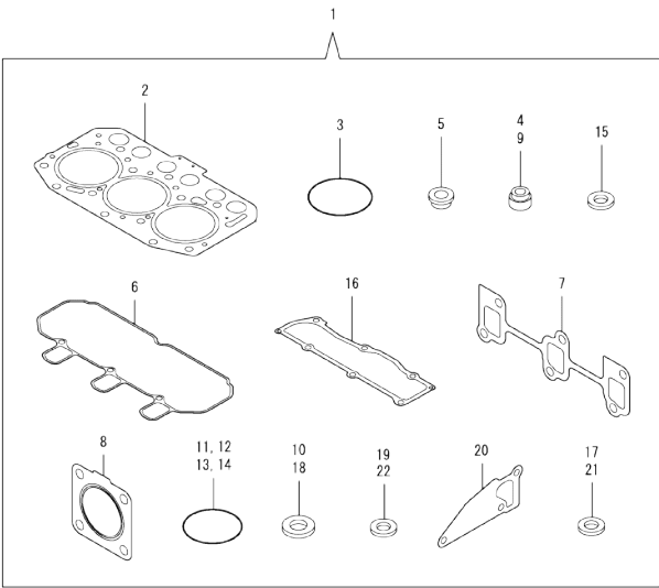
Fig.15. GASKET SET
