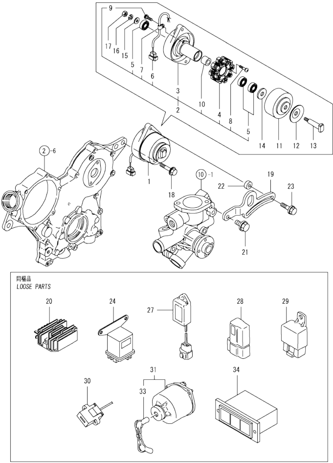
Fig.16. GENERATOR
