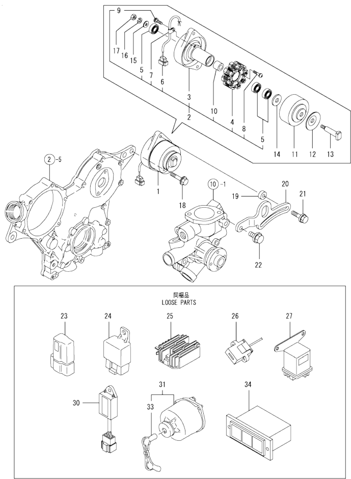
Fig.16. GENERATOR
