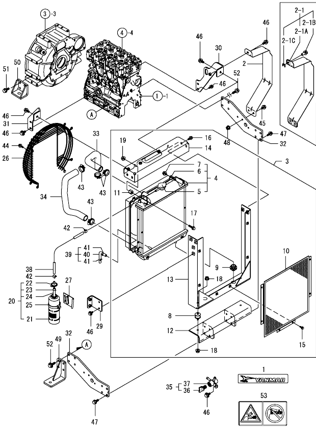
Fig.11. RADIATOR
