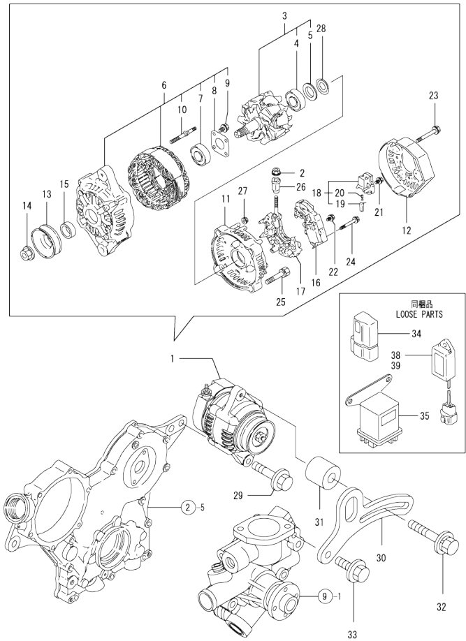
Fig.15. GENERATOR
