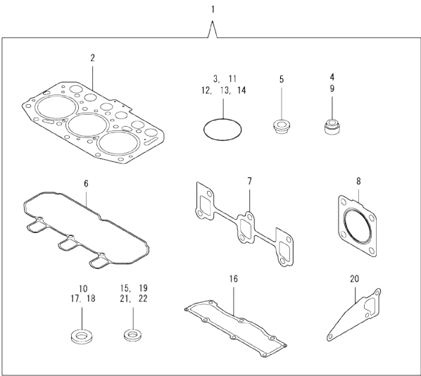
Fig.16. GASKET SET
