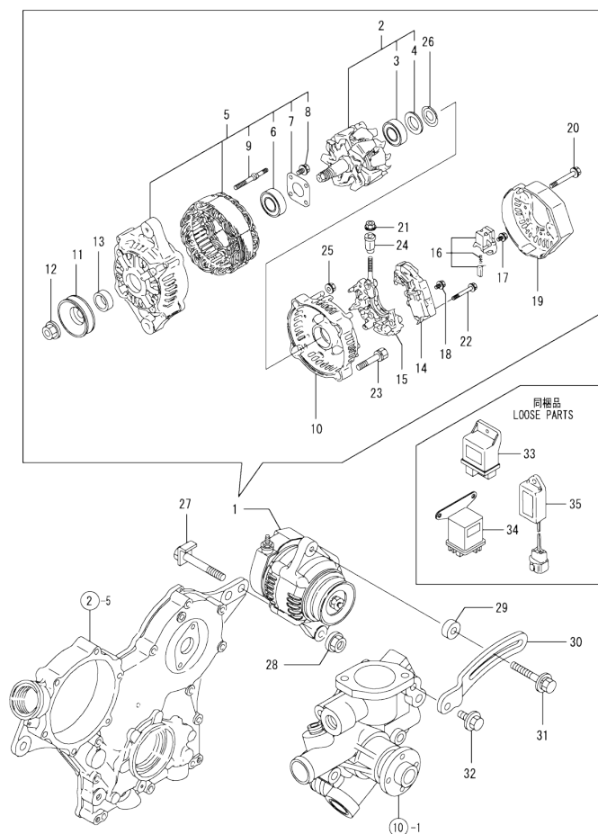
Fig.15. GENERATOR
