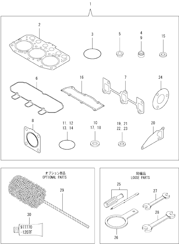
Fig.16. GASKET SET
