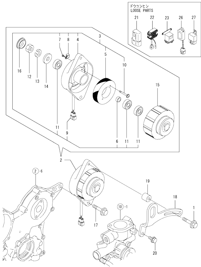
Fig.16. GENERATOR
