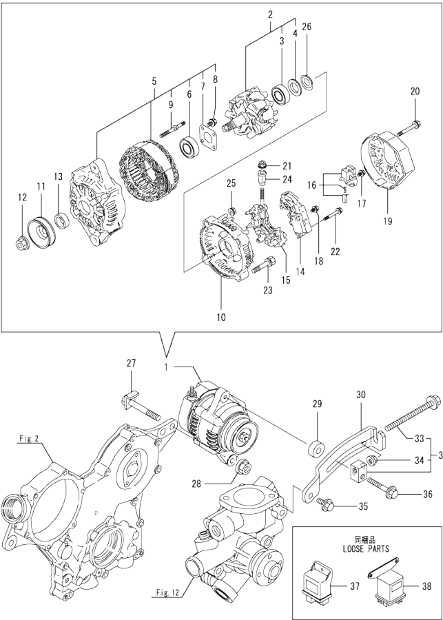
Fig.19. GENERATOR
