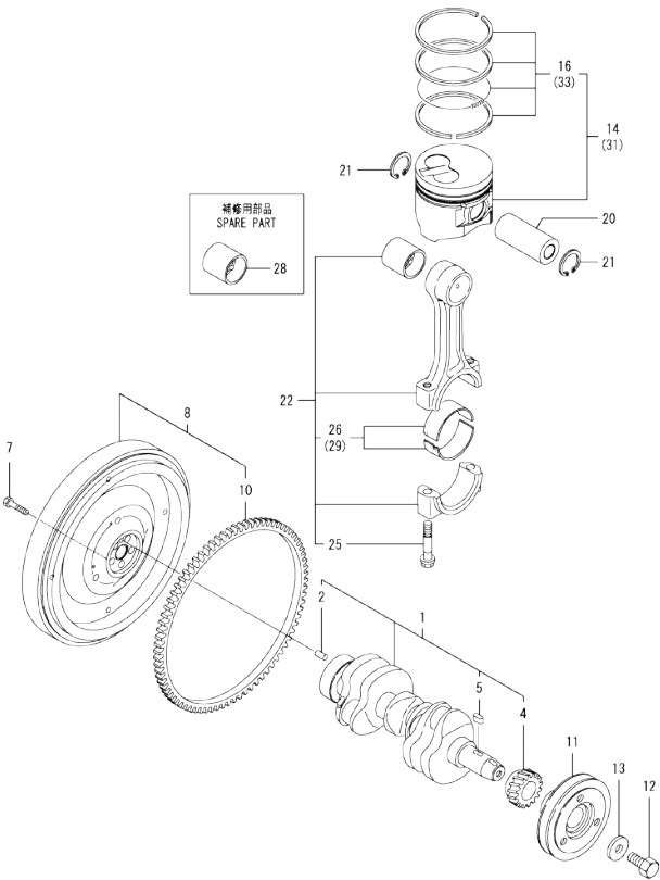
Fig.10. CRANKSHAFT & PISTON
