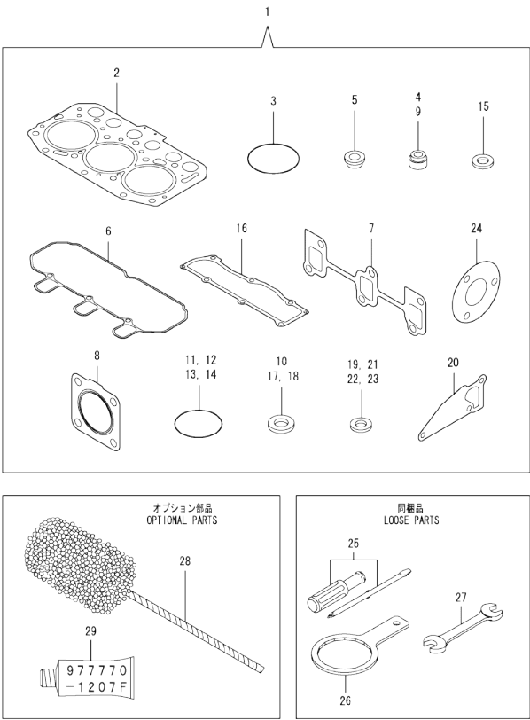
Fig.21. GASKET SET
