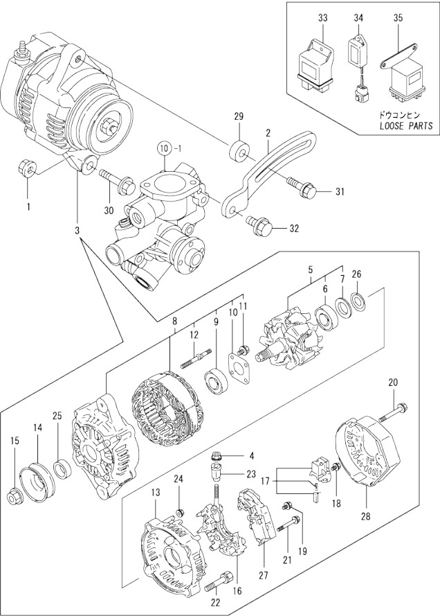
Fig.16. GENERATOR
