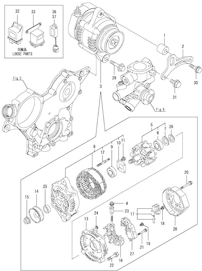
Fig.15. GENERATOR
