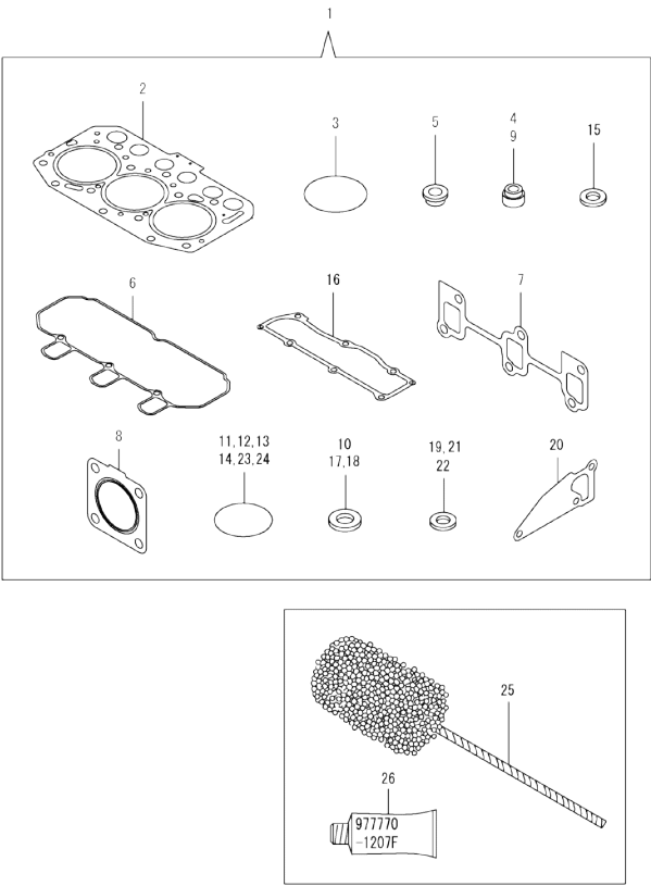
Fig.18. GASKET SET
