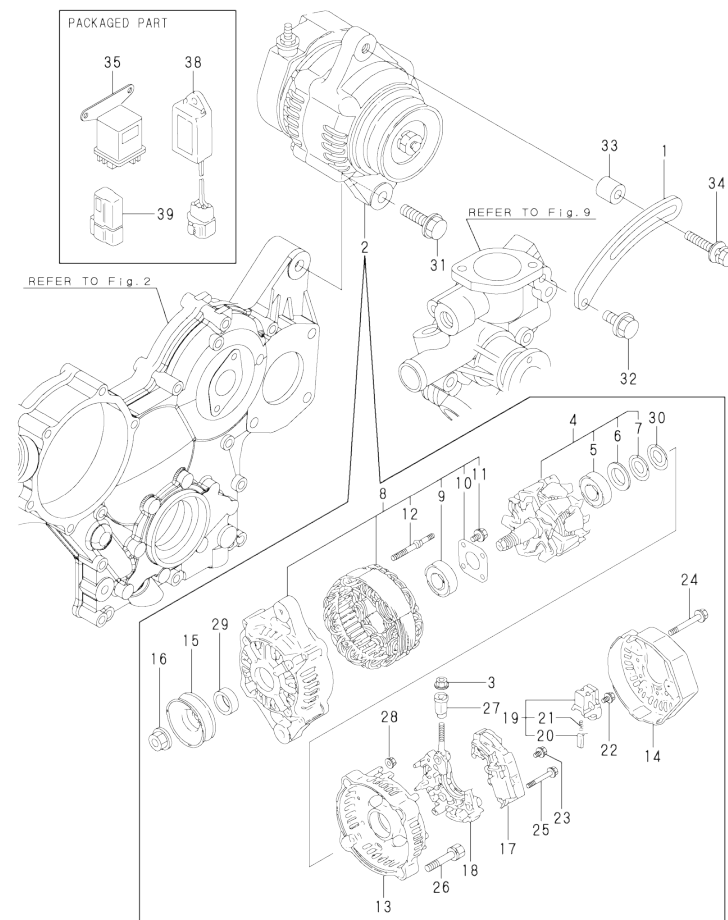
Fig.15. GENERATOR
