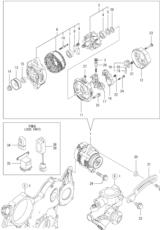
Fig.15. GENERATOR
