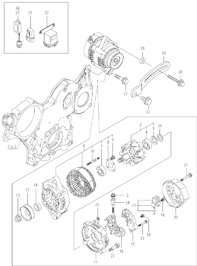
OCD50-M00050 3TNV76-DTE Fig.16. GENERATOR
