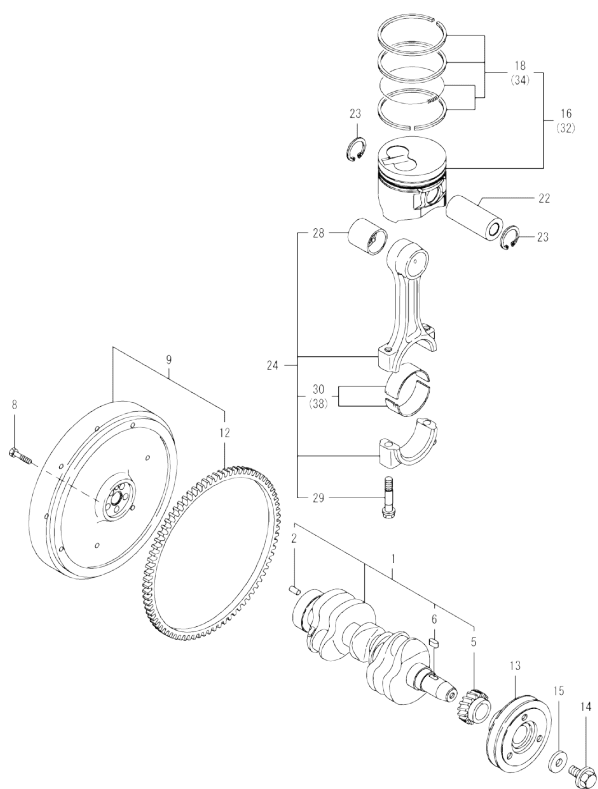
OCD50-M00050 3TNV76-DTE Fig.8. CRANKSHAFT & PISTON
