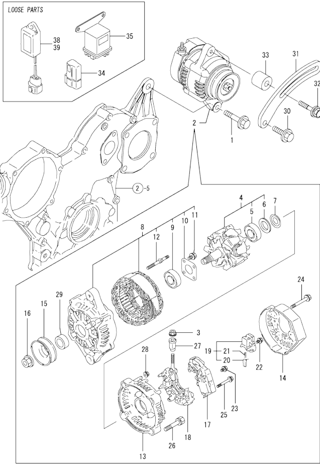
Fig.16. GENERATOR
