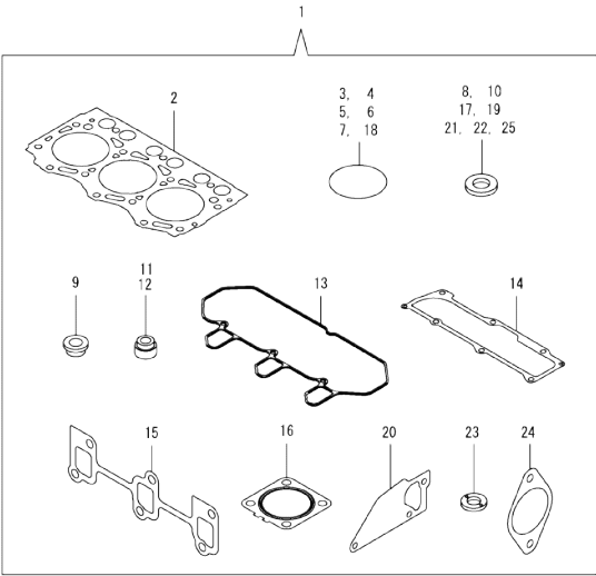
Fig.16. GASKET SET
