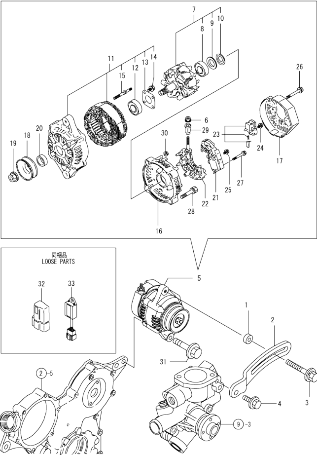
Fig.14. GENERATOR
