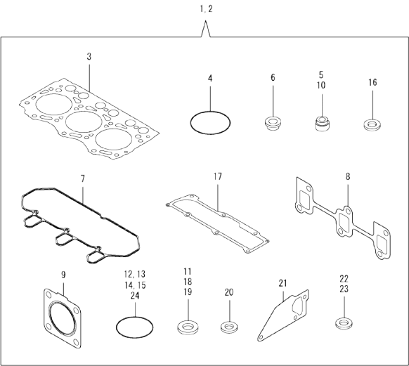
Fig.19. GASKET SET
