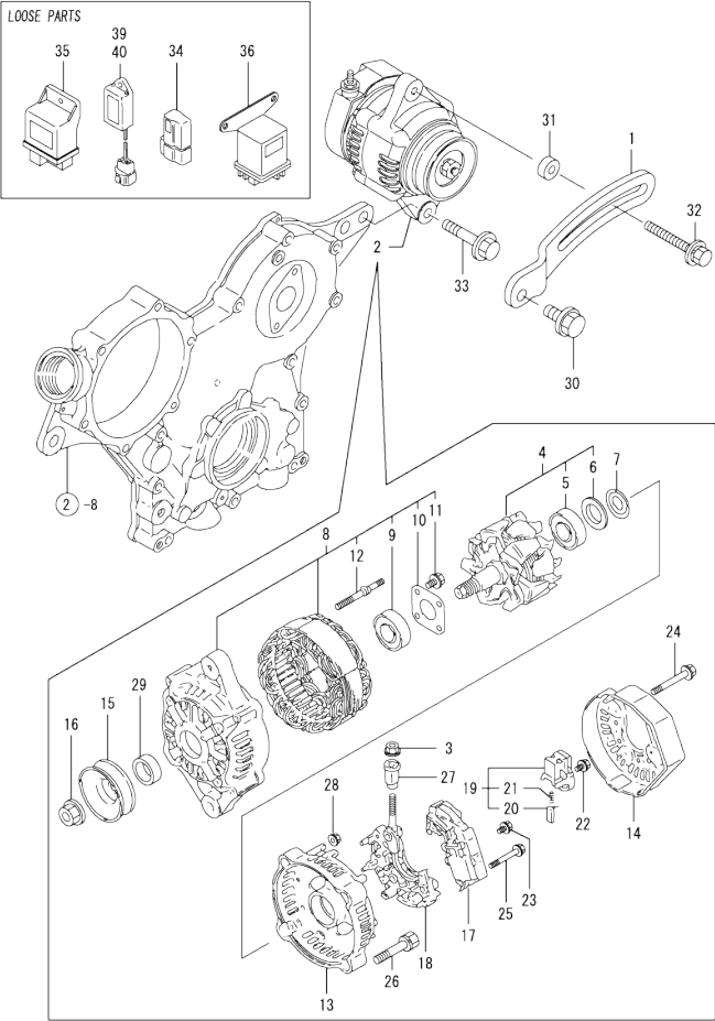
Fig.18. GENERATOR
