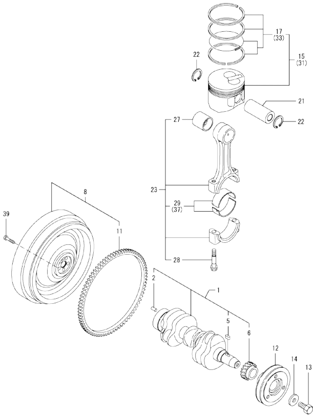
0CW10-M15900 3TNV76-GGEH Fig.8. CRANKSHAFT & PISTON
