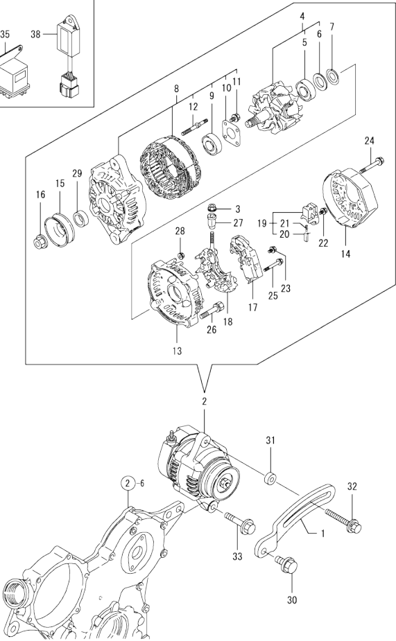
Fig.16. GENERATOR
