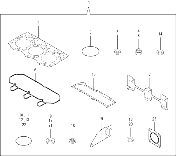
Fig.15. GASKET SET
