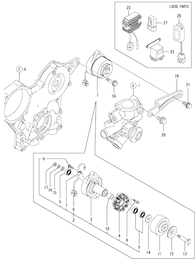
Fig.14. GENERATOR
