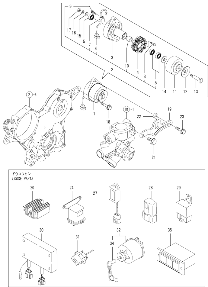
Fig.16. GENERATOR
