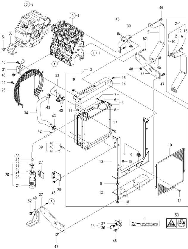
Fig.11. RADIATOR
