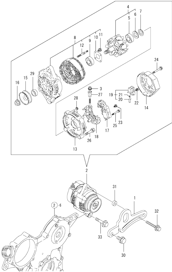
Fig.18. GENERATOR
