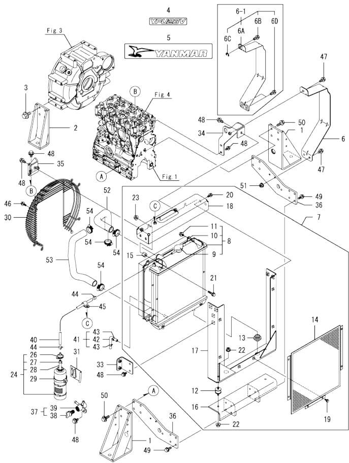
Fig.11. RADIATOR
