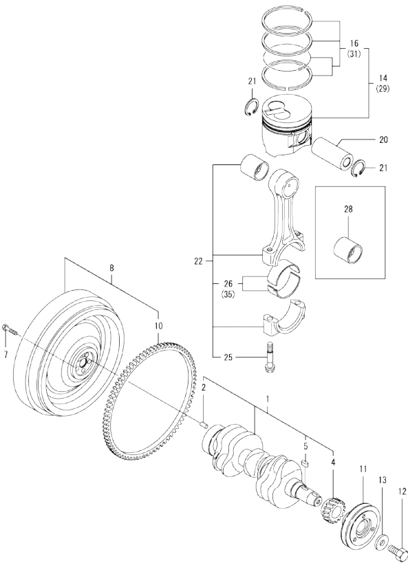
OCE10-M27001 YPU23V/YPU23V-1 Fig.8. CRANKSHAFT & PISTON
