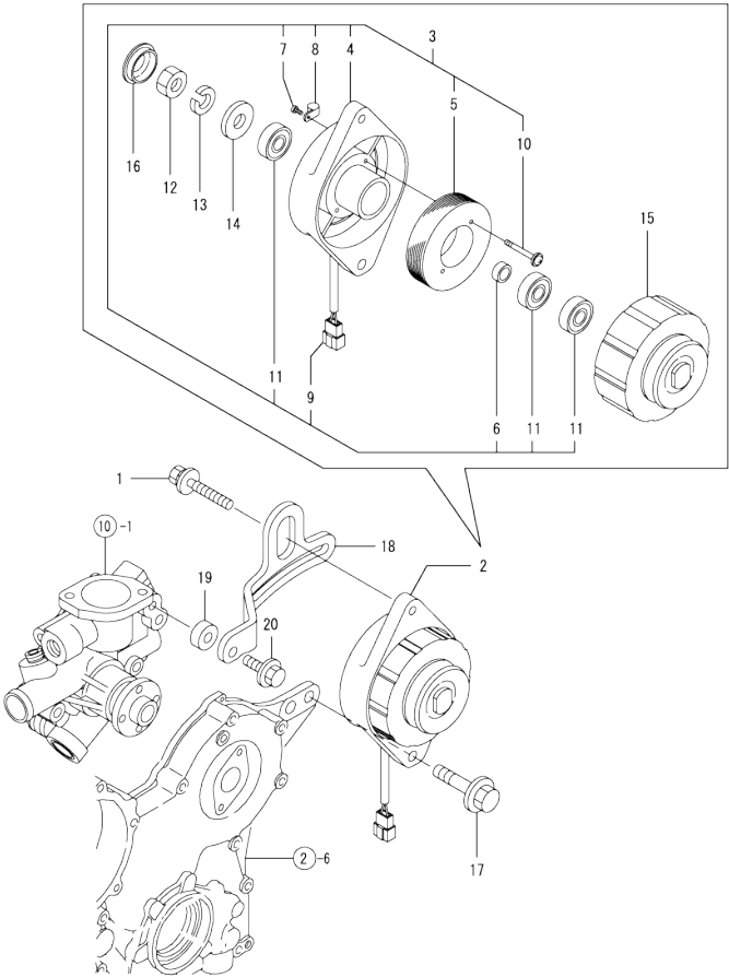
Fig.15. GENERATOR
