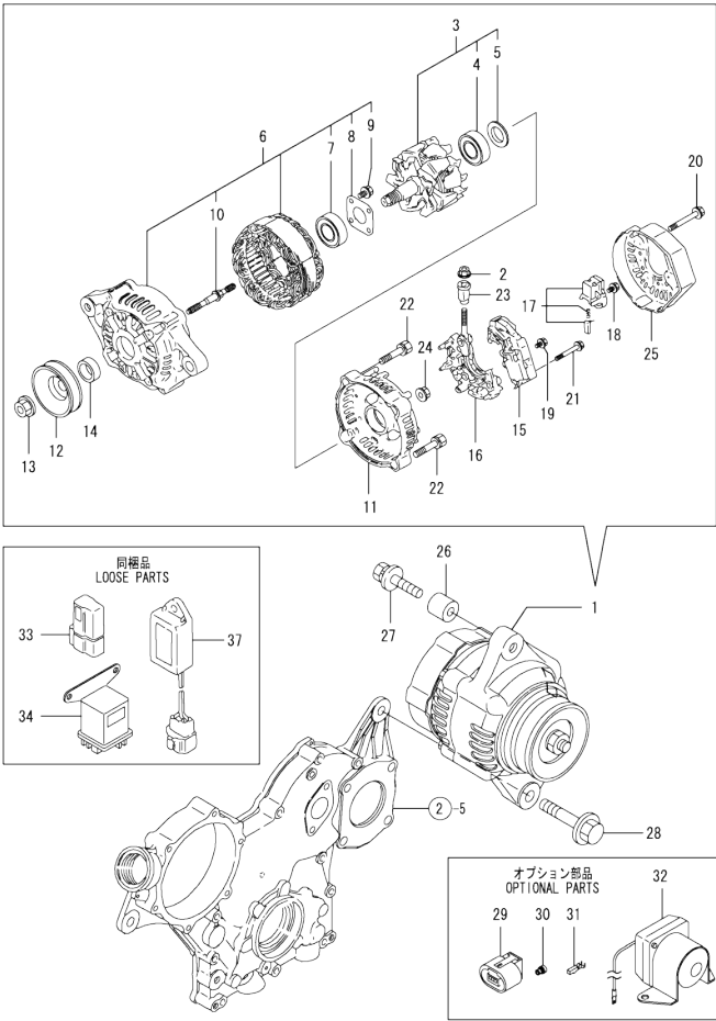
Fig.18. GENERATOR
