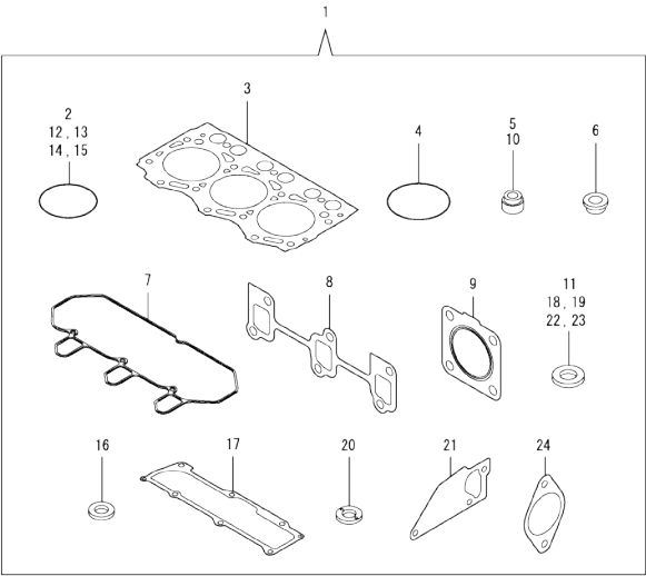
Fig.19. GASKET SET
