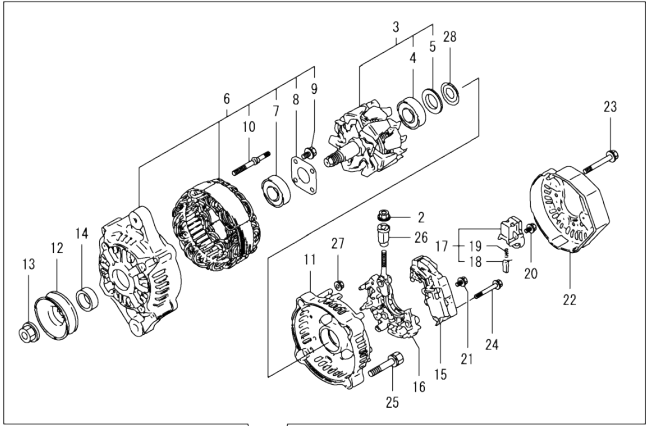
Fig.15. GENERATOR
