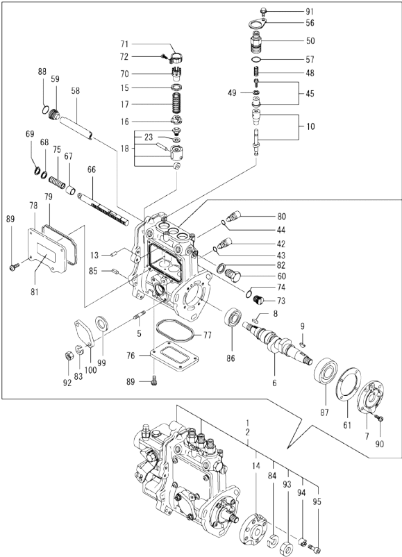
OCD10-M81601 3TNV76-SIK/QIK Fig.10. FUEL INJECTION PUMP
