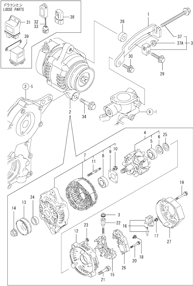
Fig.15. GENERATOR
