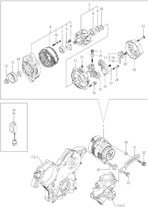
Fig.15. GENERATOR
