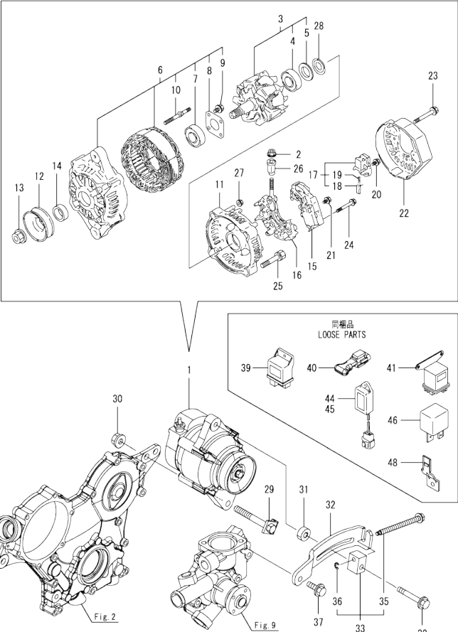
Fig.15. GENERATOR
