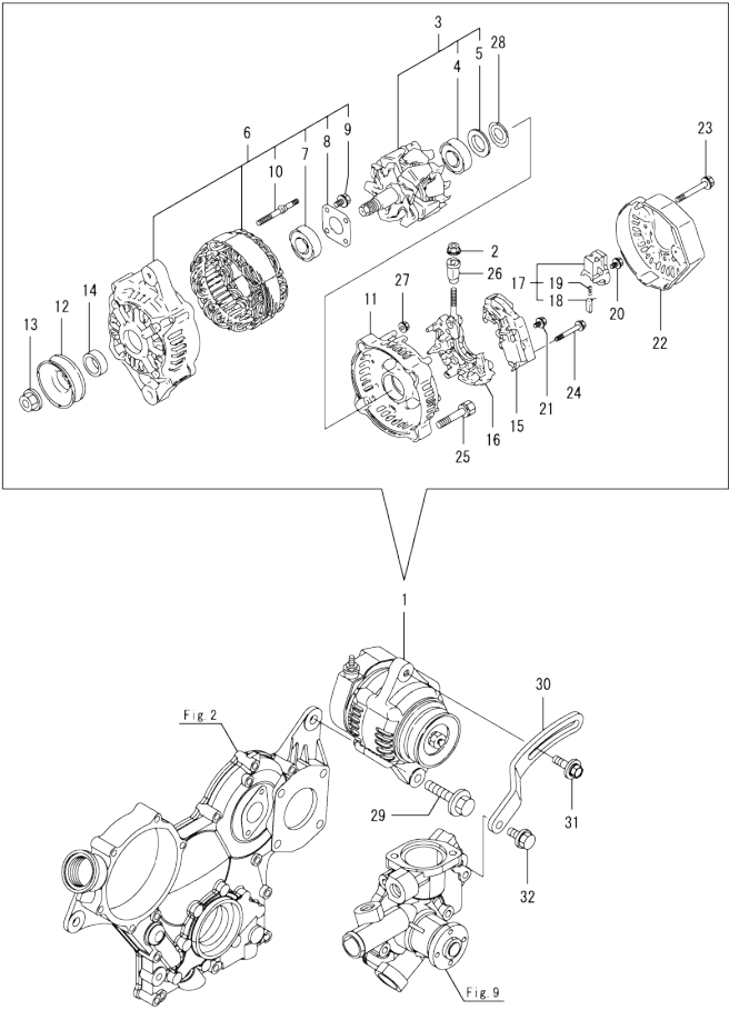
Fig.15. GENERATOR
