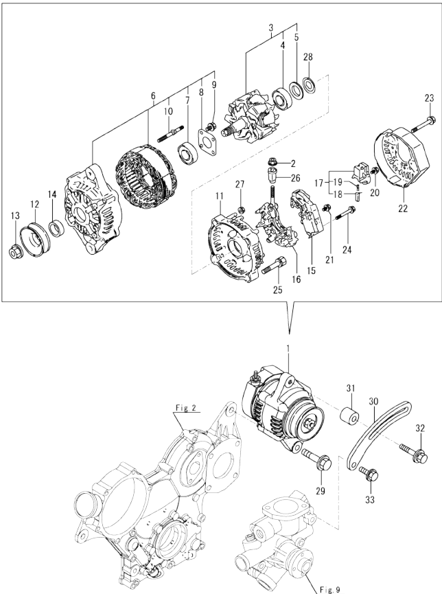
Fig.15. GENERATOR
