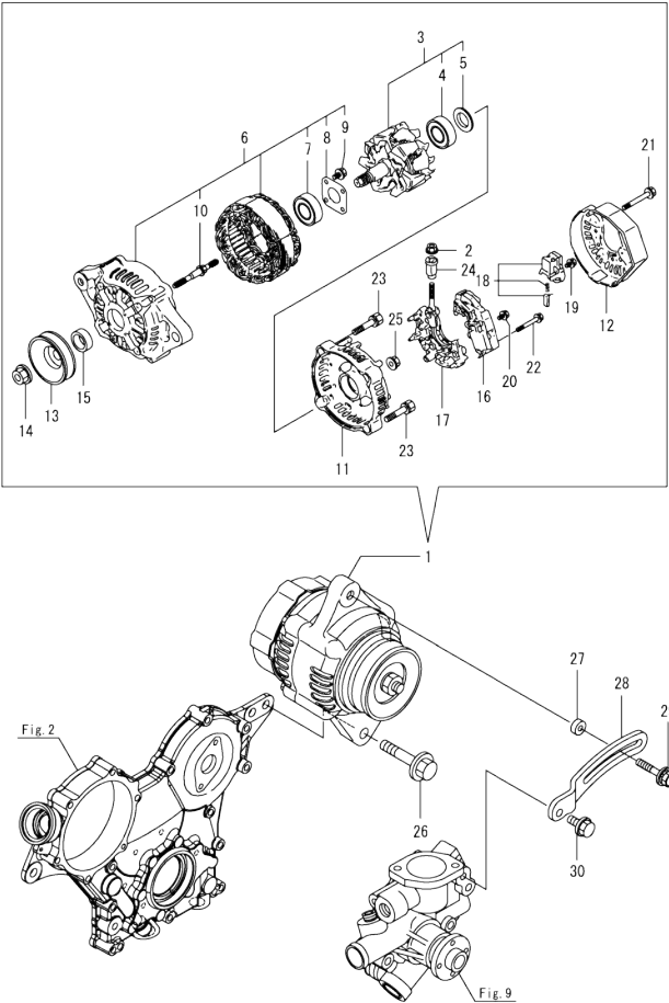
Fig.15. GENERATOR
