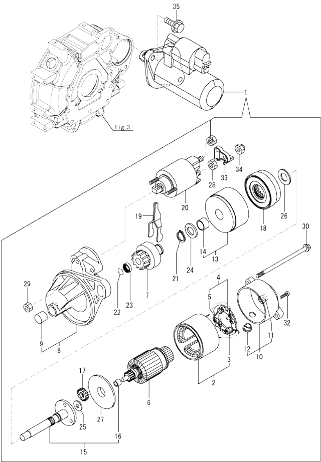
Fig.16. STARTER MOTOR
