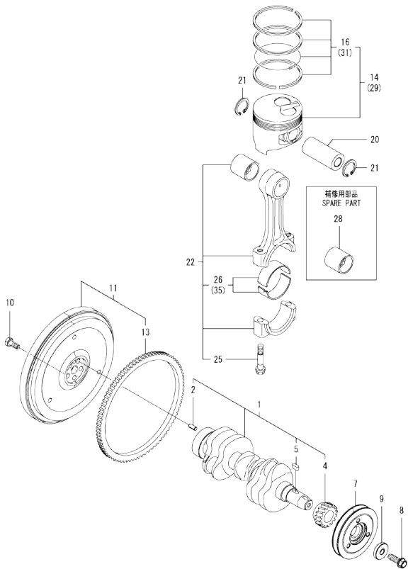
OCD50-M01160 3TNV76-XPAZ Fig.8. CRANKSHAFT & PISTON
