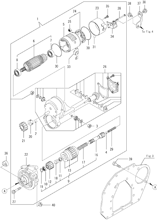
Fig.16. (14A)STARTER MOTOR
