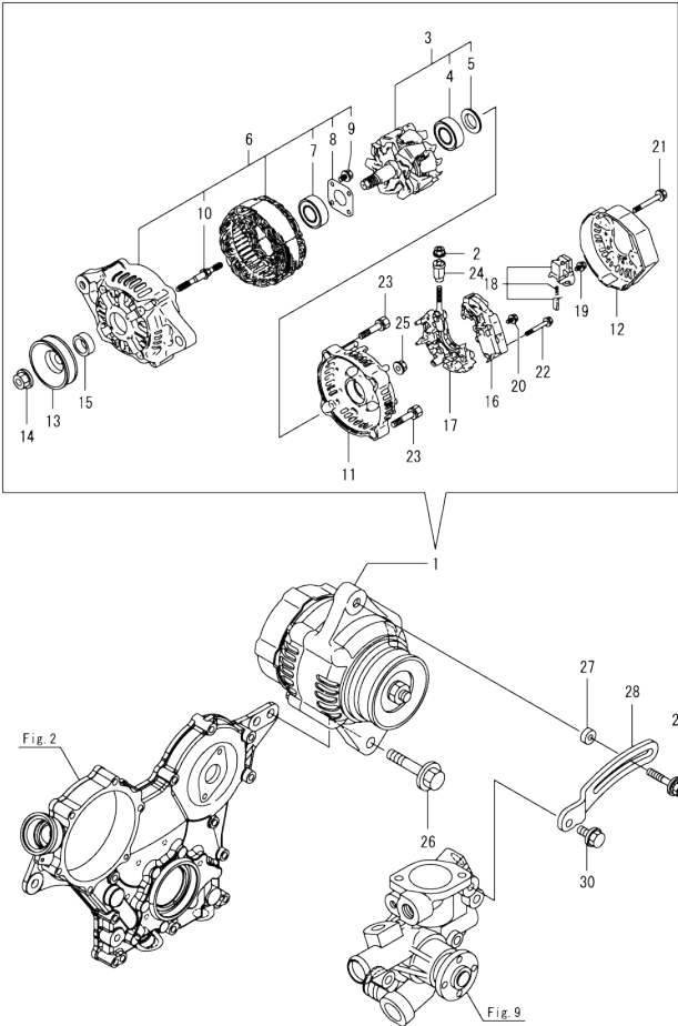
Fig.15. GENERATOR
