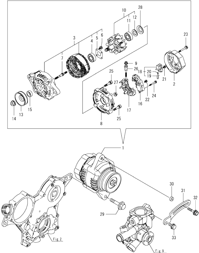
Fig.14. GENERATOR
